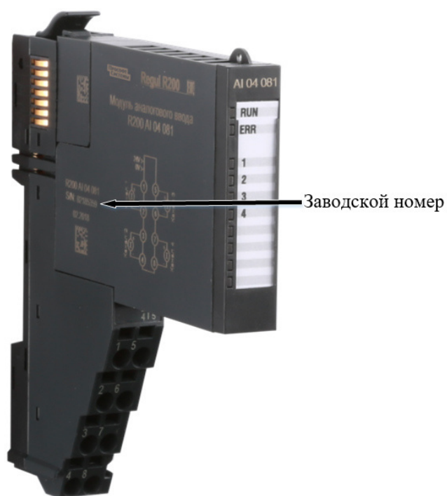
Рисунок 1 – Общий вид модулей REGUL R200
