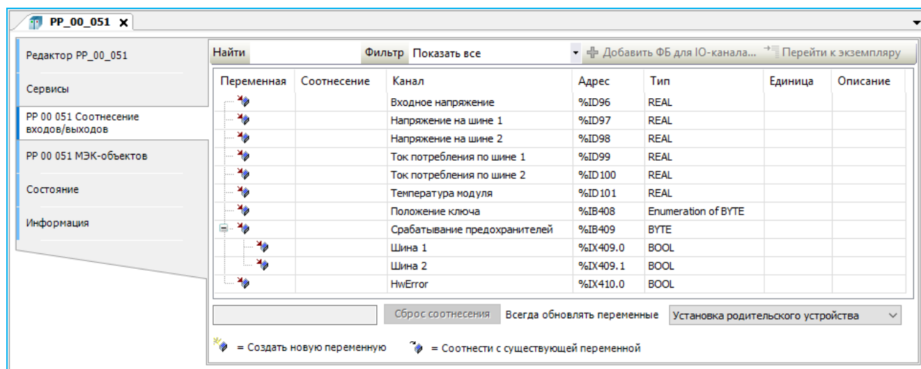
Рисунок 127 - Модуль источника питания R500 PP 00 051
