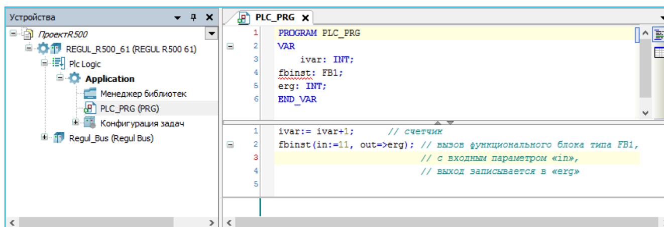
Рисунок 169 – Пример ввода программного кода
