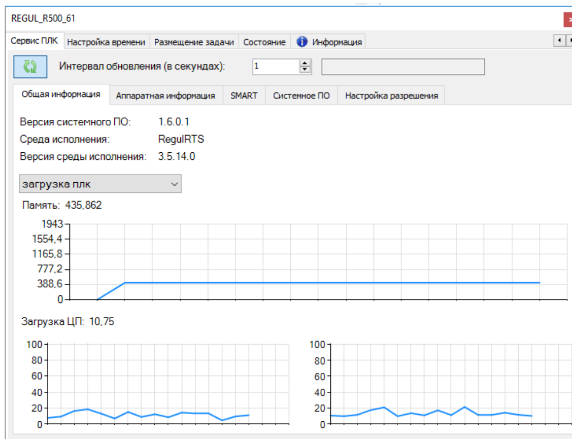
Рисунок 199 – Пример данных по загрузке ПЛК
