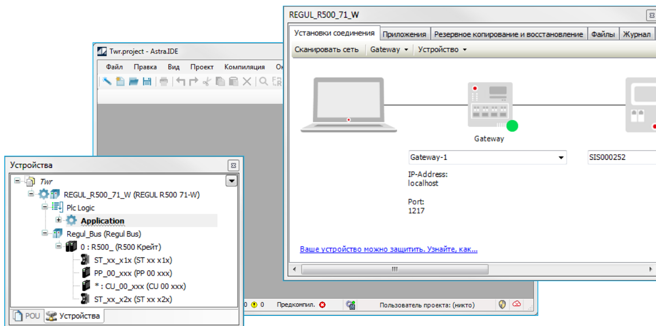
Рисунок 18 – Окна и вкладки в виде отдельных окон
