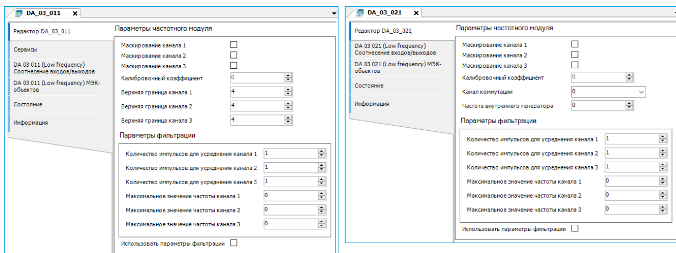
Рисунок 111 – Параметры каналов модулей на примере модуля R500 DA 03 011 и модуля R600 DA 03 021
