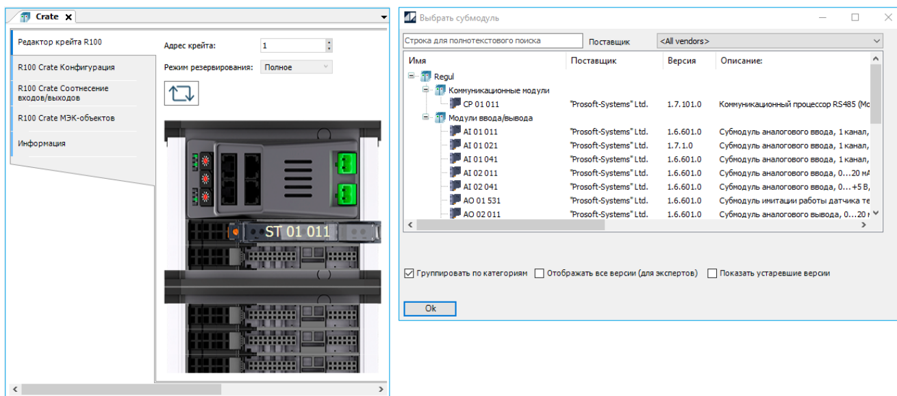
Рисунок 73 - Добавление submodule в крейт R100
