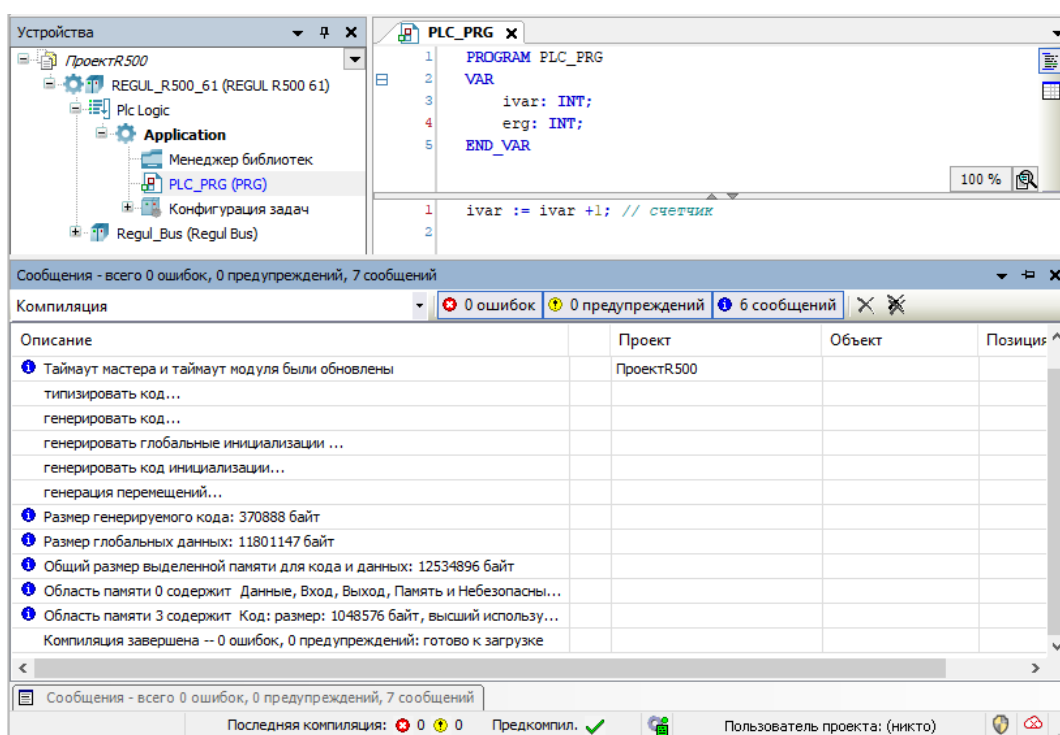
Рисунок 172 – Окно сообщений. Компиляция завершена
