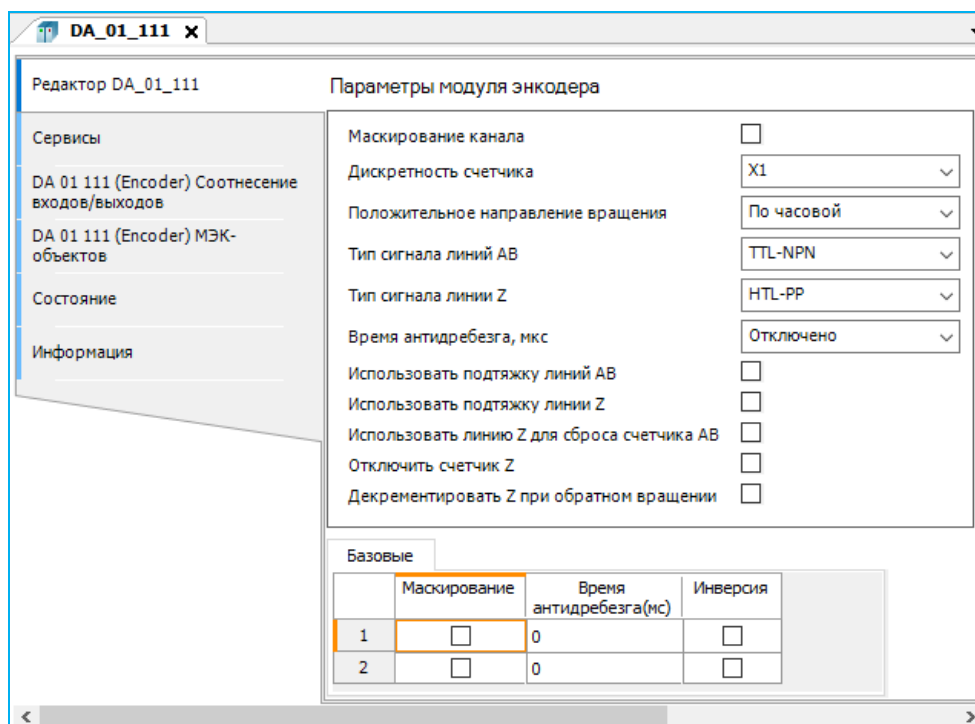
Рисунок 113 – Параметры каналов модуля счета импульсов R200 DA 01 111
