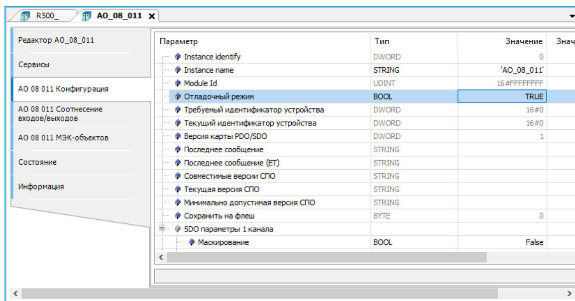
Рисунок 206 – Включение отладочного режима для модуля
