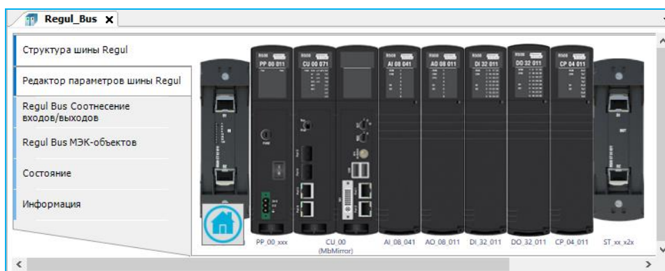
Рисунок 47 – Редактор шины контроллера R500
