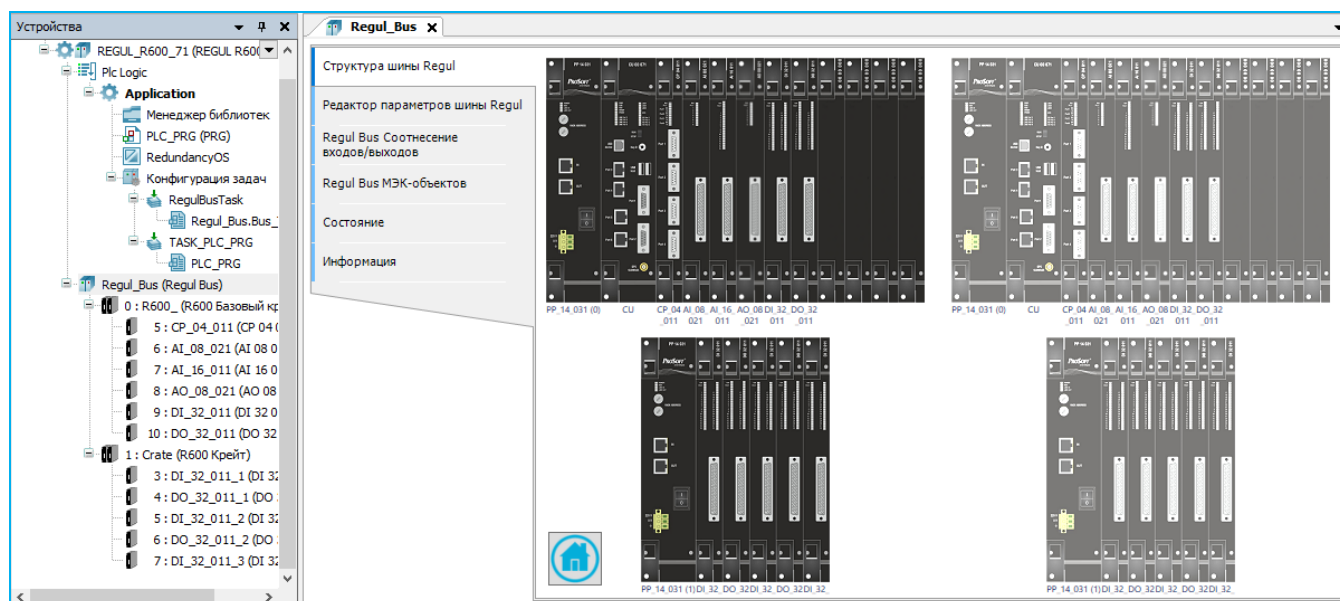
Рисунок 50 – Структура шины контроллера R600 (2 крейта, с полным резервированием)
