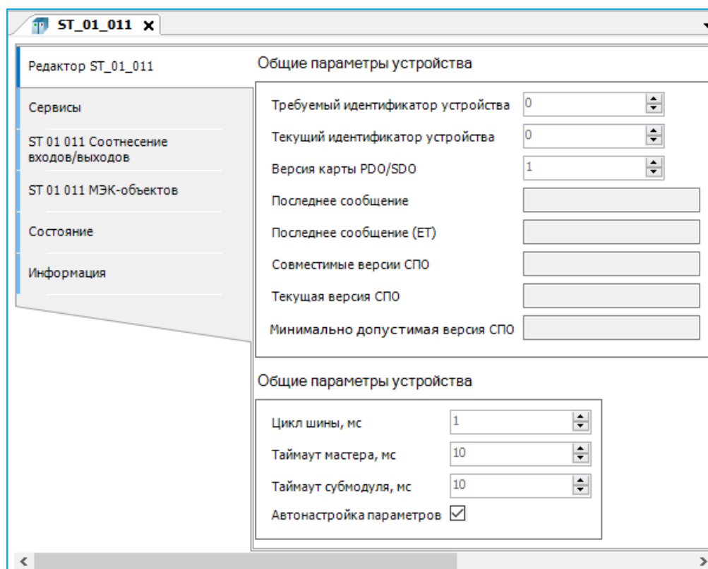
Рисунок 56 – Настраиваемые параметры внутренней шины крейта R100
