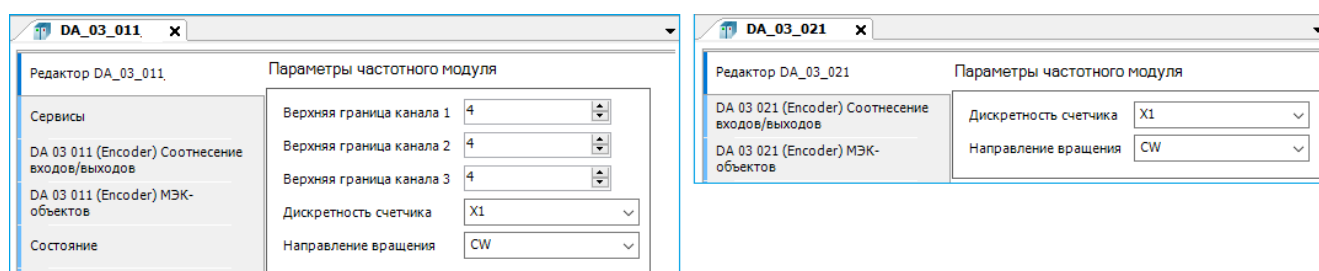
Рисунок 112 – Параметры каналов модулей на примере модуля R500 DA 03 011 и модуля R600 DA 03 021
