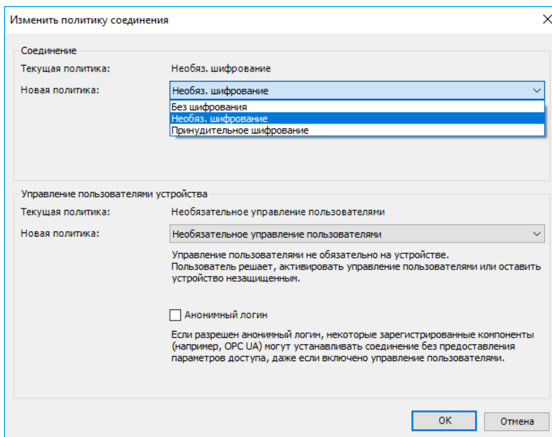
Рисунок 163 – Окно изменения политики соединения
