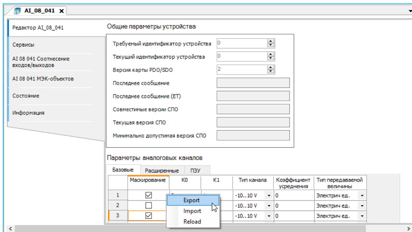
Рисунок 88 – Контекстное меню для сохранения/восстановления настроек
