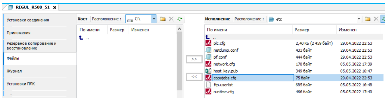
Рисунок 195 – Конфигурационный файл расположенный в папке etc на контроллере
