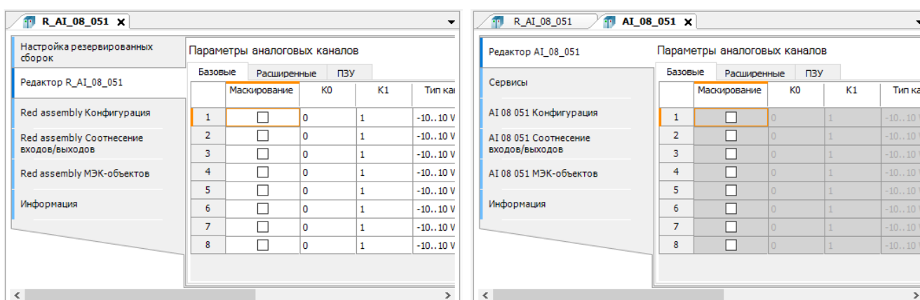
Рисунок 82 – Редактор параметров аналоговых каналов модуля для резервированной сборки на примере модуля аналогового ввода AI 08 051
