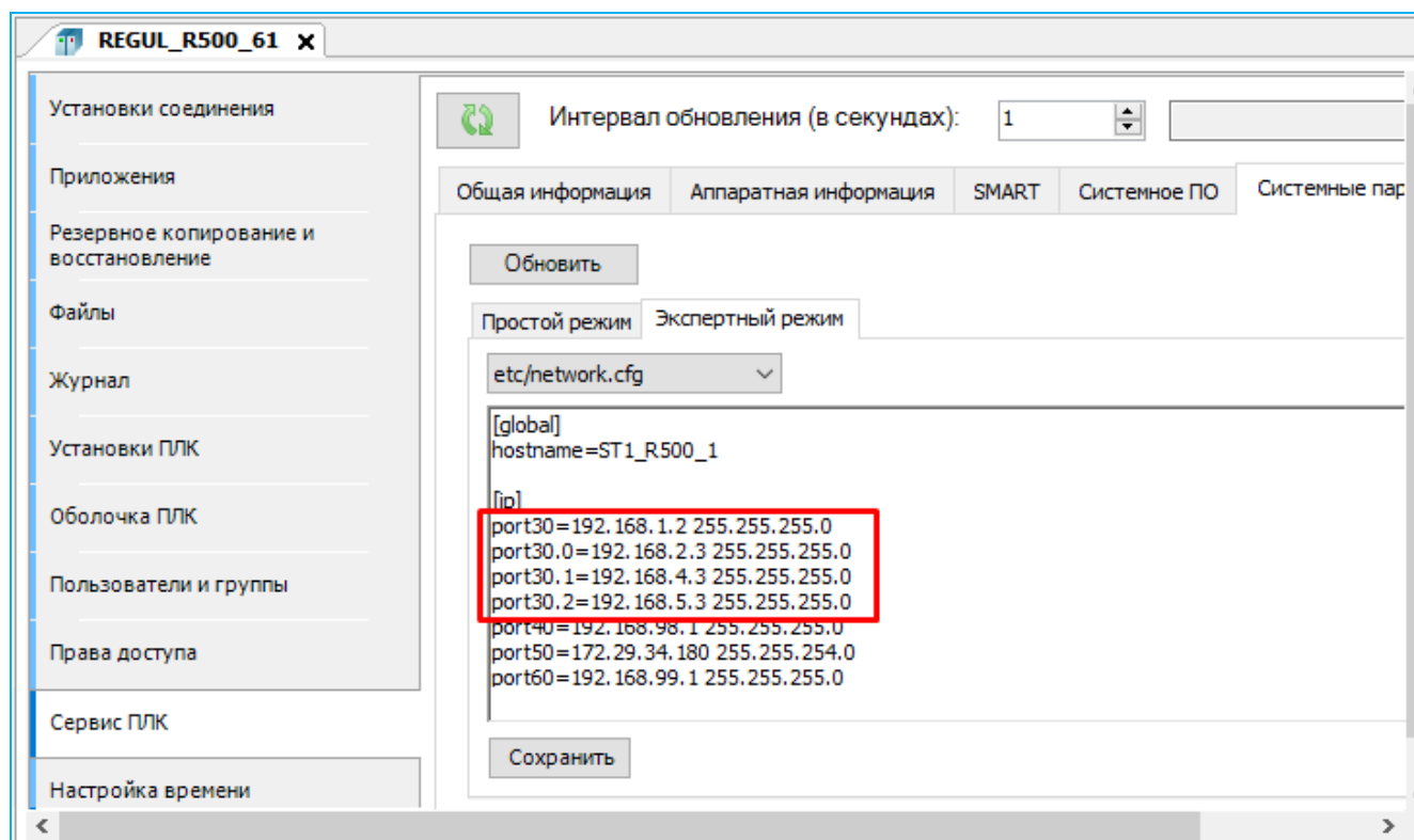
Рисунок 145 – Установка дополнительных IP-адресов
