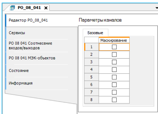
Рисунок 90 – Базовые параметры модуля R500 PO 08 041
