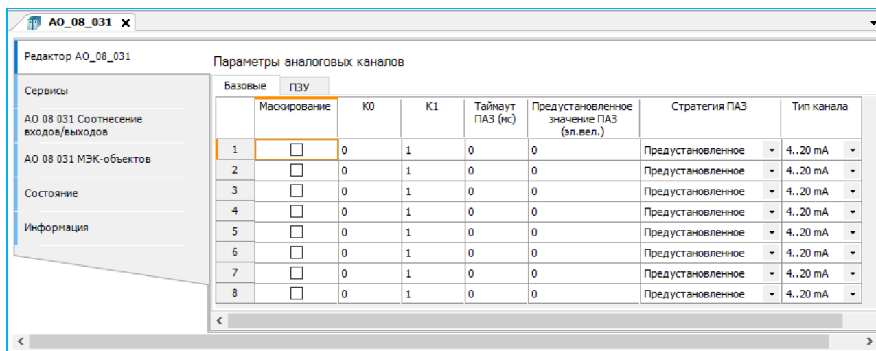
Рисунок 99 – Базовые параметры аналоговых каналов на примере модуля R500 AO 08 031
