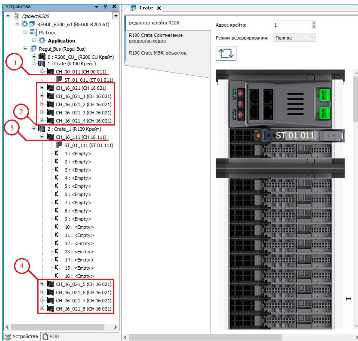
Рисунок 72 – Редактор крейтов контроллера Regul R100
