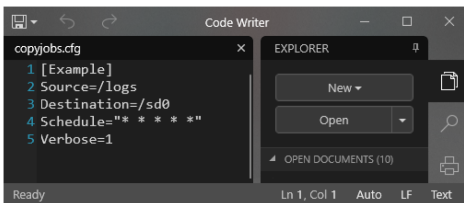
Рисунок 196 – Конфигурационный файл copyjobs.cfg
