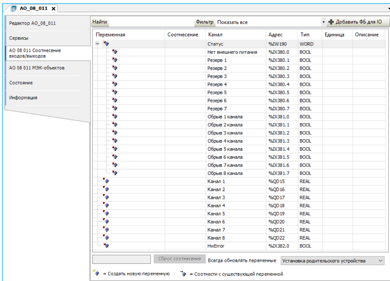
Рисунок 126 – Проверка статуса модуля аналогового вывода
