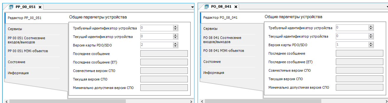
Рисунок 89 - Пример отображения редактора модуля R500 PP 00 051 и R500 PO 08 041
