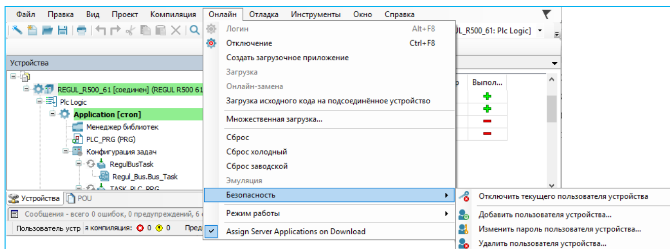
Рисунок 268 – Диалоговое окно управления онлайн - пользователями
