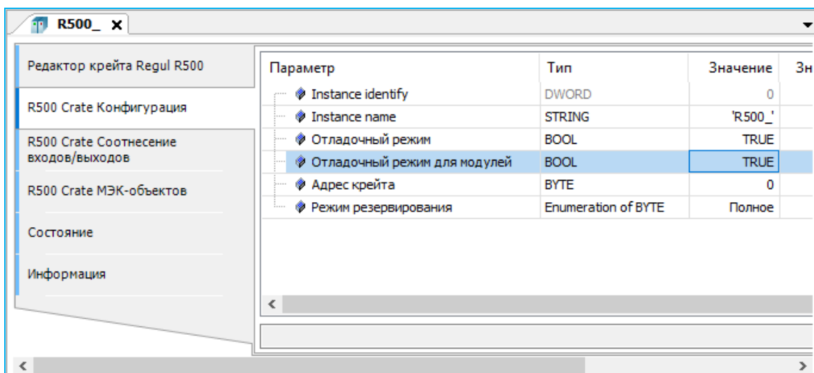
Рисунок 205 – Включение отладочного режима для всех модулей
