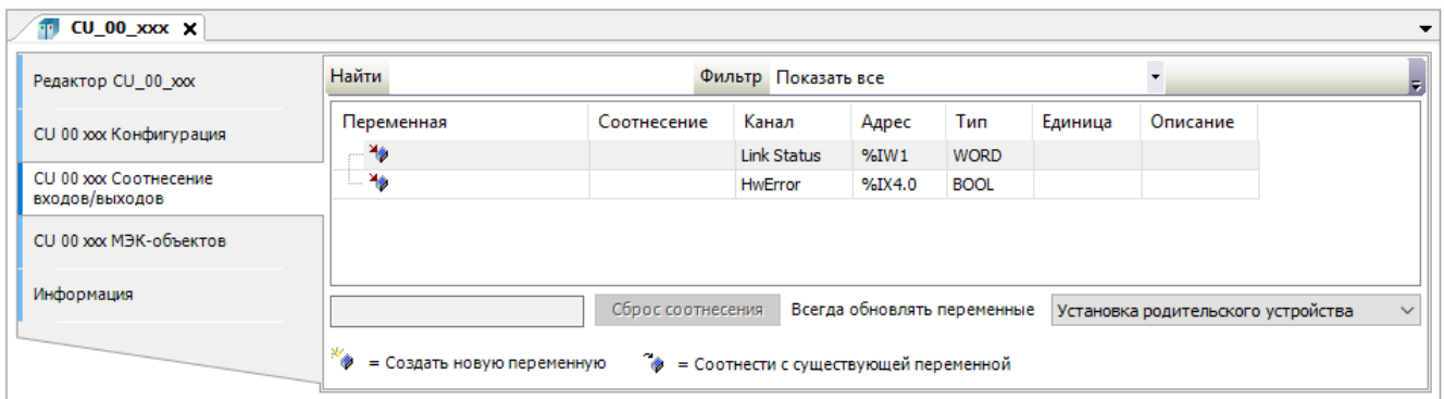
Рисунок 130 – Пример вкладки соотнесение входов/выходов модулей ЦП III-го типа
