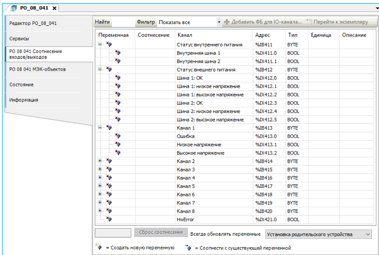
Рисунок 128 - Модуль источника внешнего питания R500 PO 08 041
