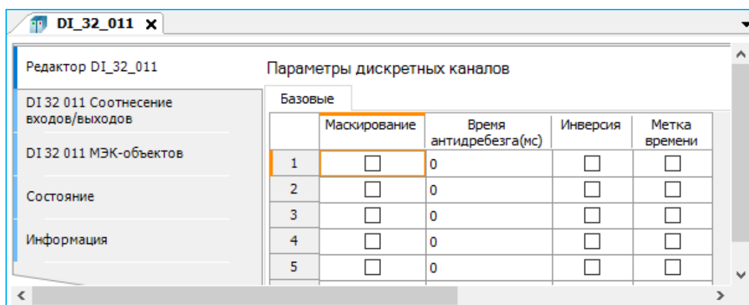
Рисунок 102 – Параметры дискретных каналов на примере модуля R600 DI 32 011
