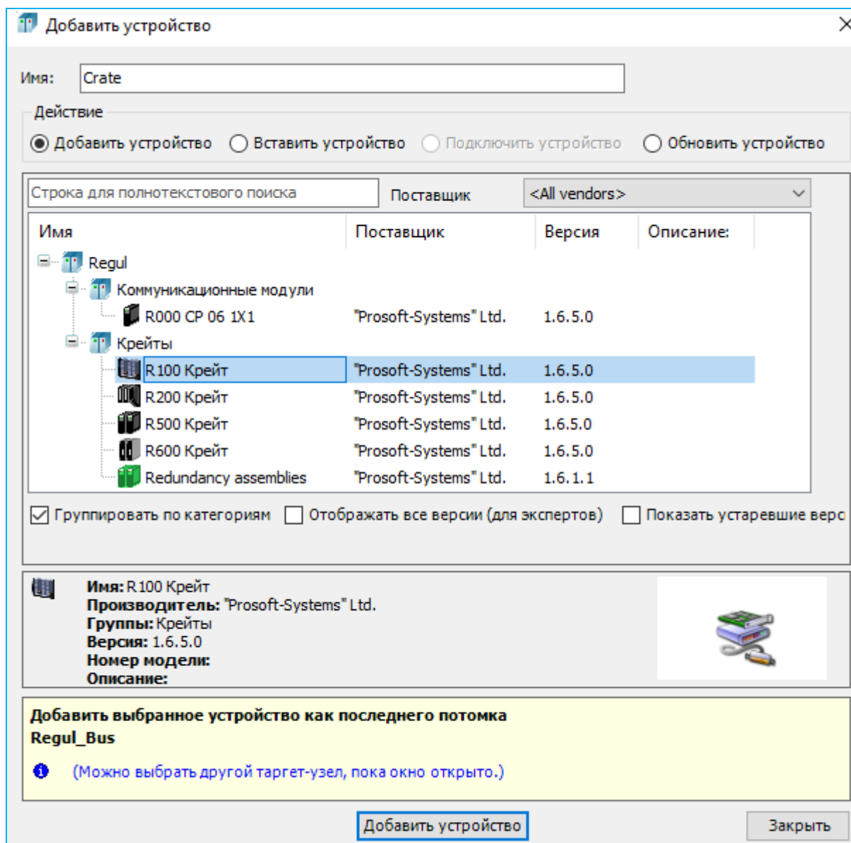
Рисунок 44 – Добавление крейта на внутреннюю шину RegulBus
