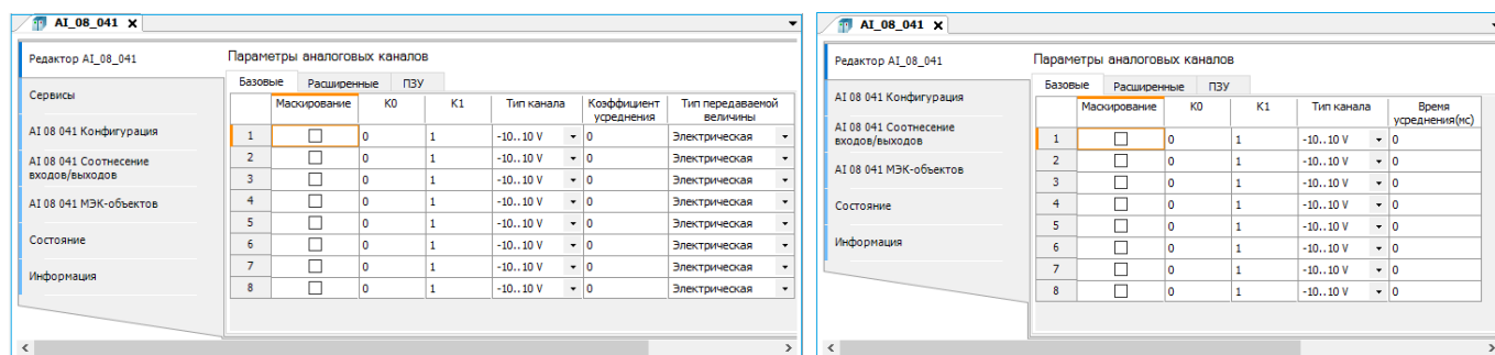
Рисунок 92 – Базовые параметры аналоговых каналов на примере модуля R500 AI 08 041 и модуля R600 AI 08 041
