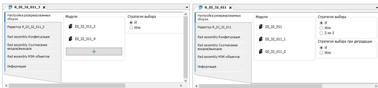
Рисунок 80 - Конфигурирование резервированных сборок модулей дискретного ввода
