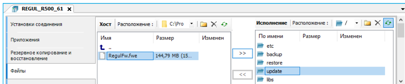
Рисунок 247– Копирование файла системного ПО на контроллер (OS QNX)
