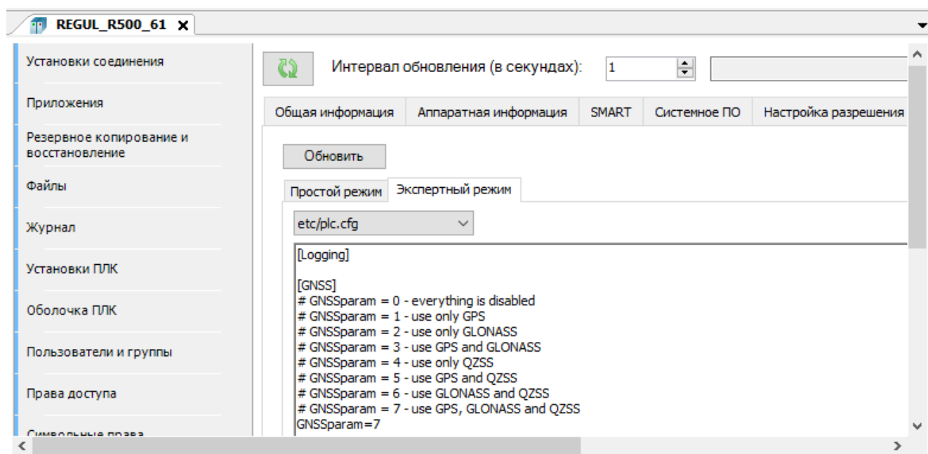
Рисунок 221 – Возможность блокировки сигналов точного времени от спутников
