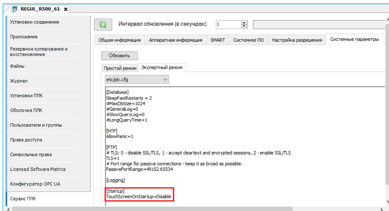
Рисунок 234 – Отключение сенсорного экрана контроллера на время загрузки
