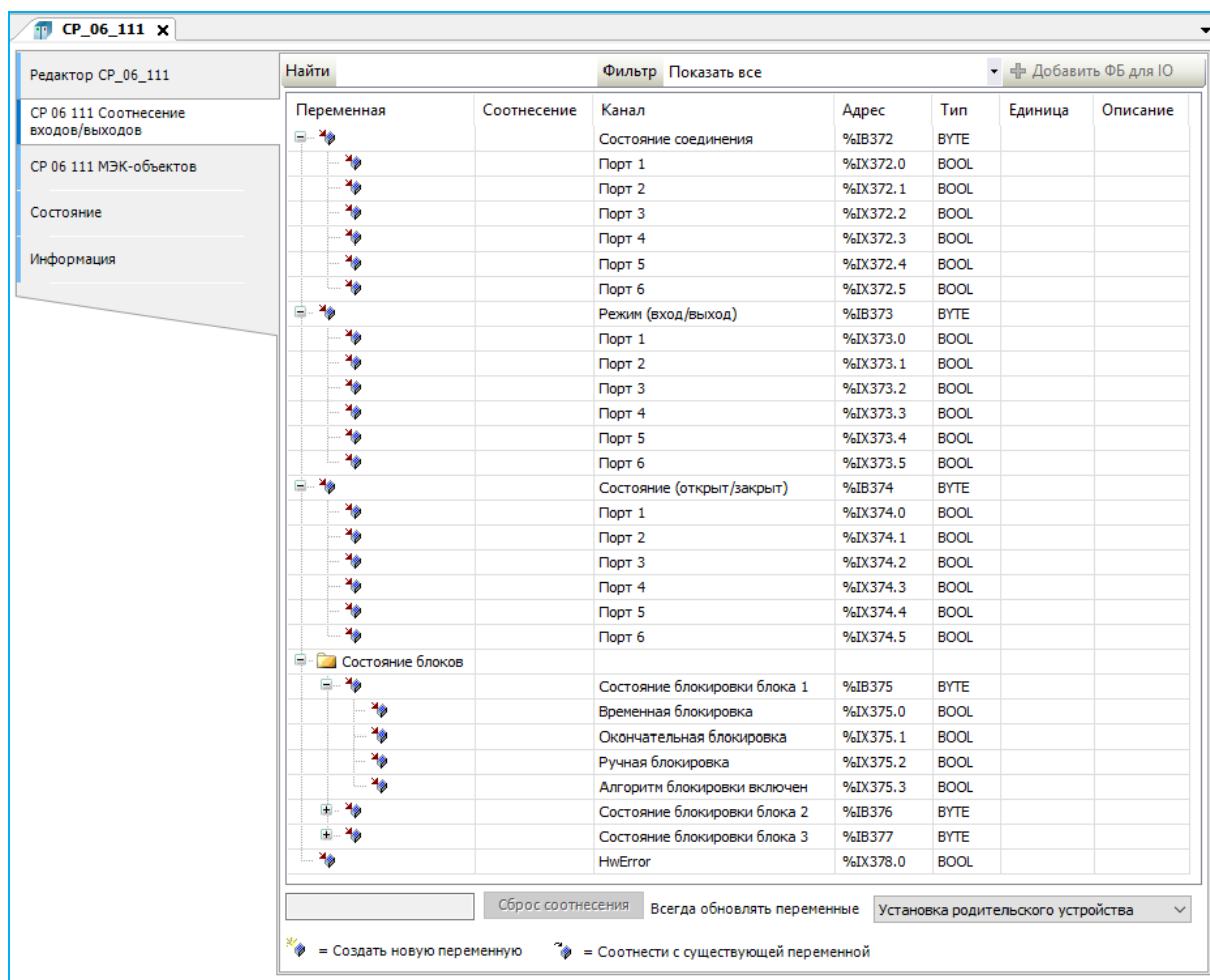
Рисунок 119 – Вкладка соотнесение входов/выходов на примере модуля CP 06 111
