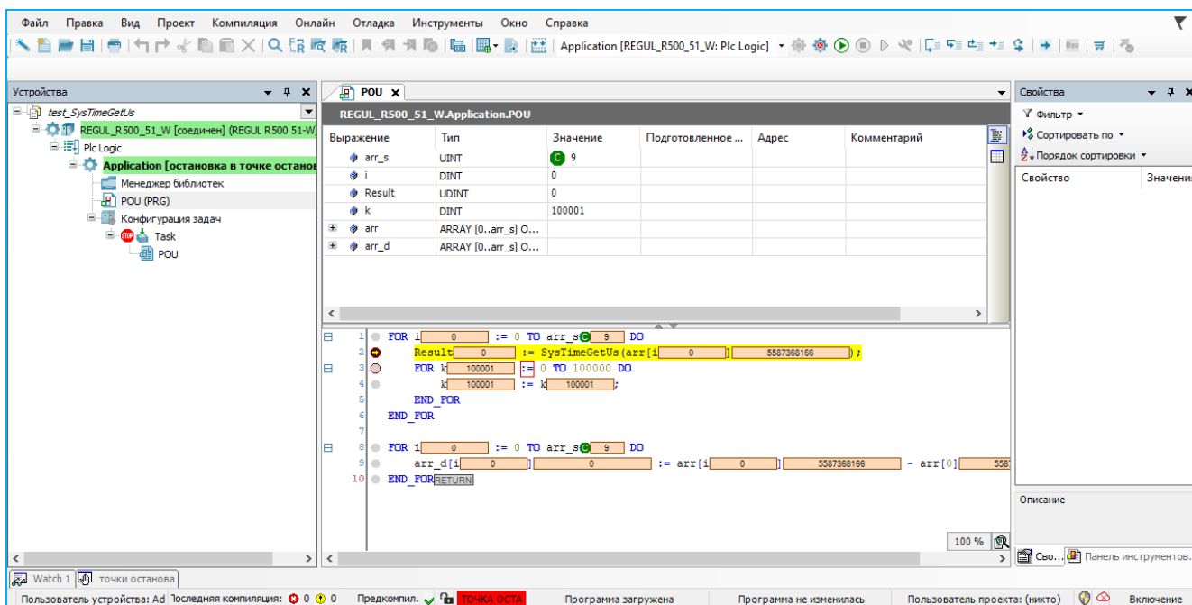
Рисунок 182 – Точка останова в ПЛК-программе
