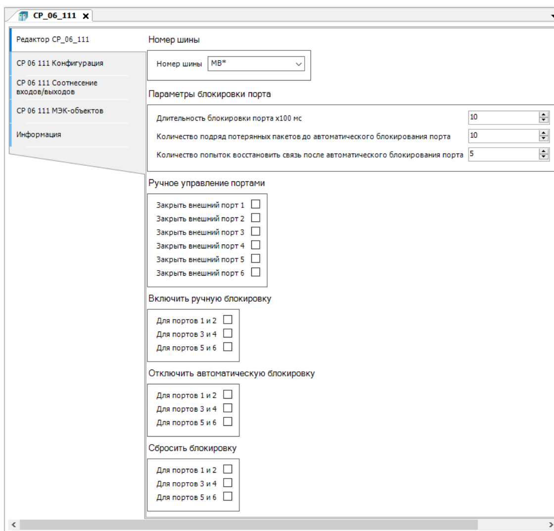
Рисунок 118 – Параметры коммуникационного модуля R500 CP 06 111 (аналогично для Regul R000 CP 06 1X1)
