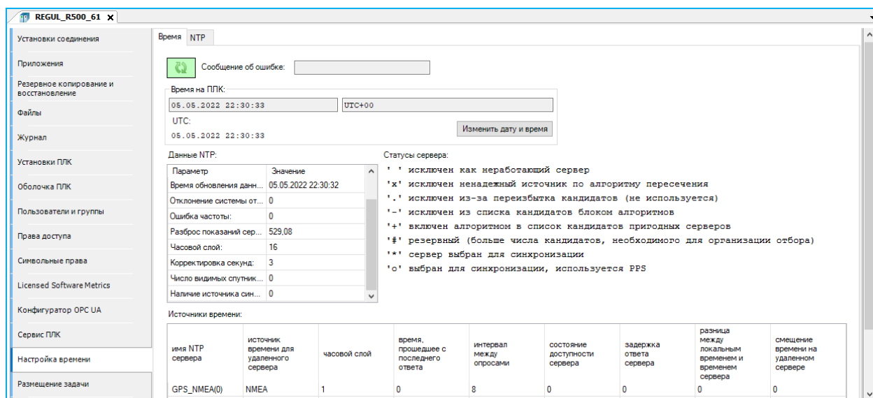
Рисунок 216 – Просмотр и настройка установок времени контроллера
