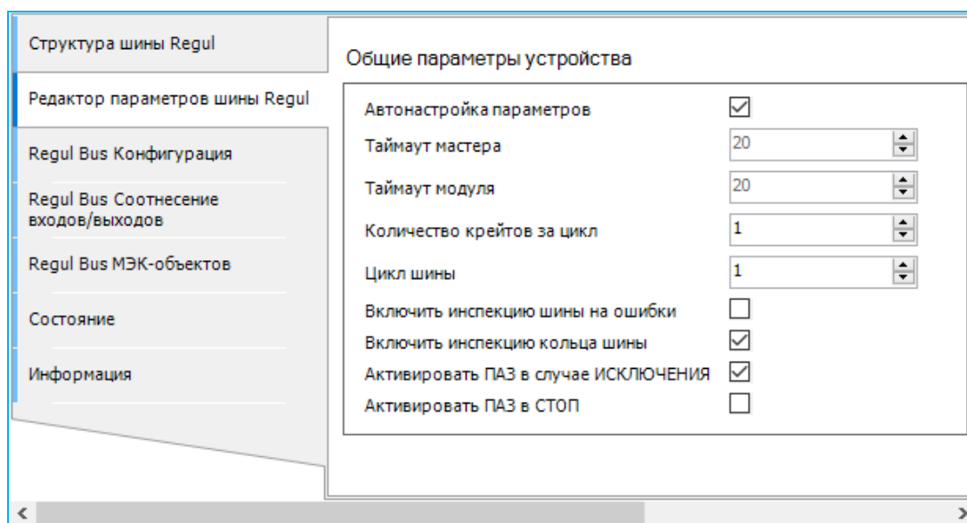
Рисунок 53 – Редактор параметров шины RegulBus OS
