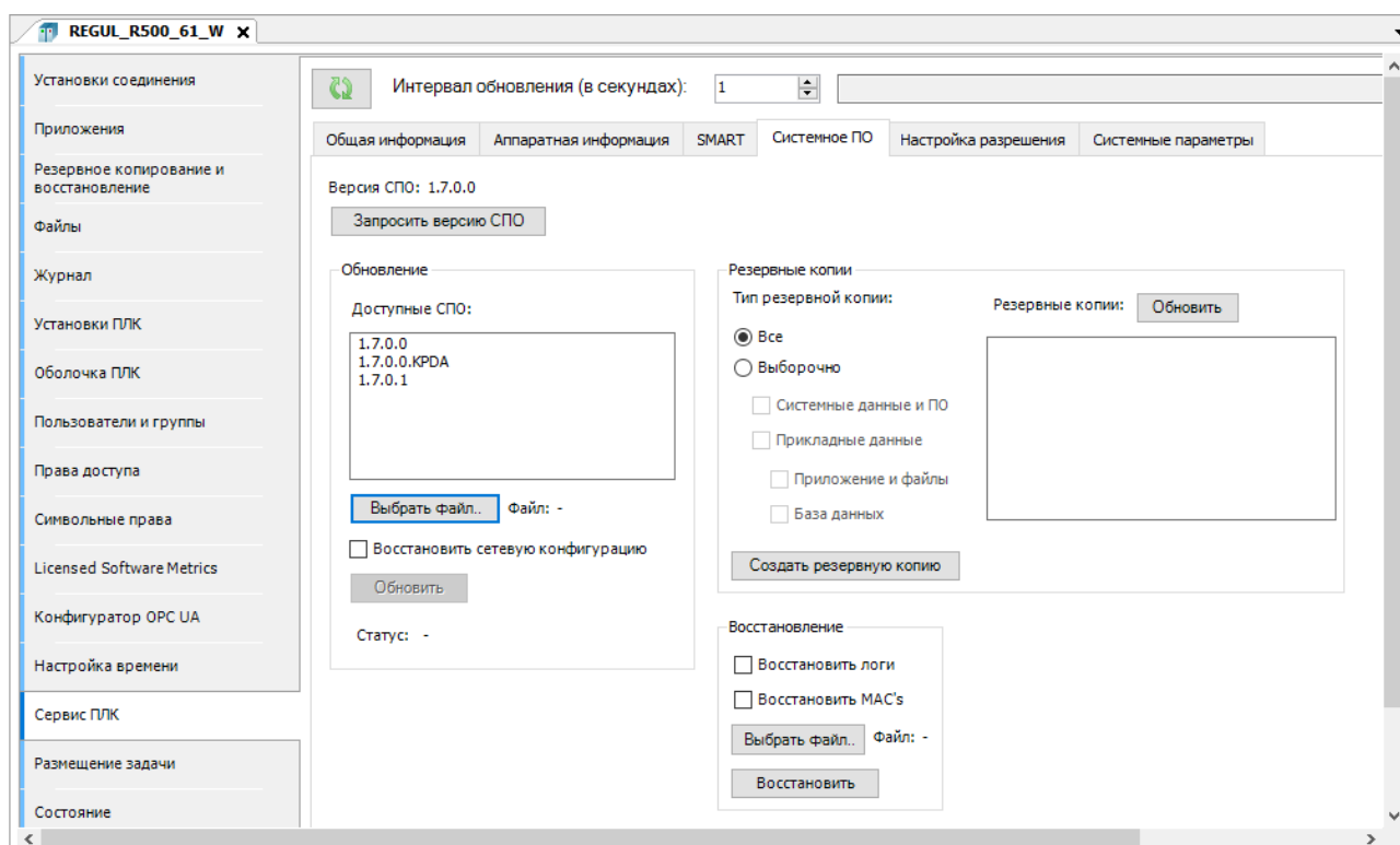
Рисунок 235 – Резервное копирование и восстановление
