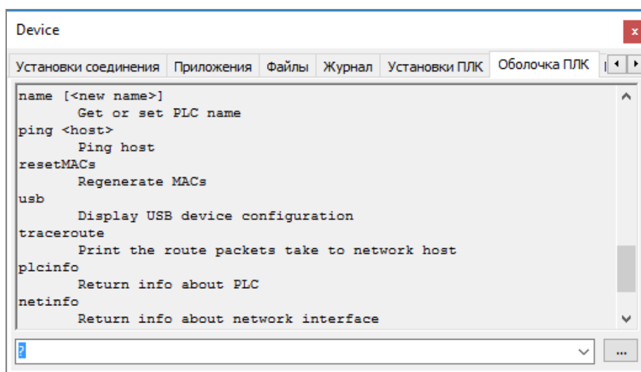
Рисунок 167 – Команды для диагностики маршрутов
