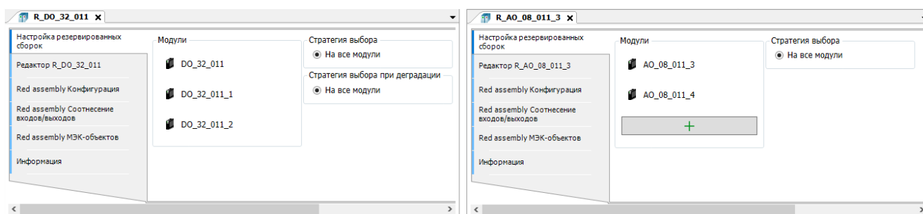
Рисунок 81 - Вкладка Настройка резервированных сборок модулей аналогового/дискретного вывода
