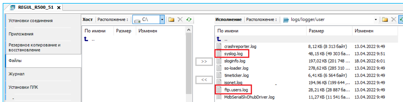
Рисунок 188 – Расположение лог-файлов на контроллере
