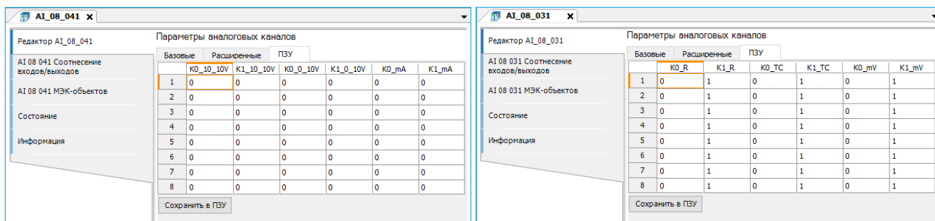
Рисунок 98 – Установка калибровочных коэффициентов каналов на примере модулей R600 AI 08 041 и R600 AI 08 031
