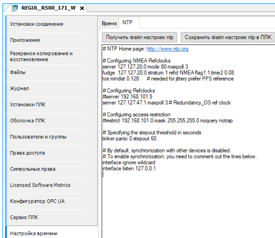
Рисунок 220 – Редактирование настроек NTP
