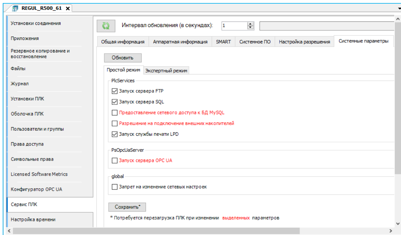
Рисунок 184 – Вкладка с системными параметрами в простом режиме
