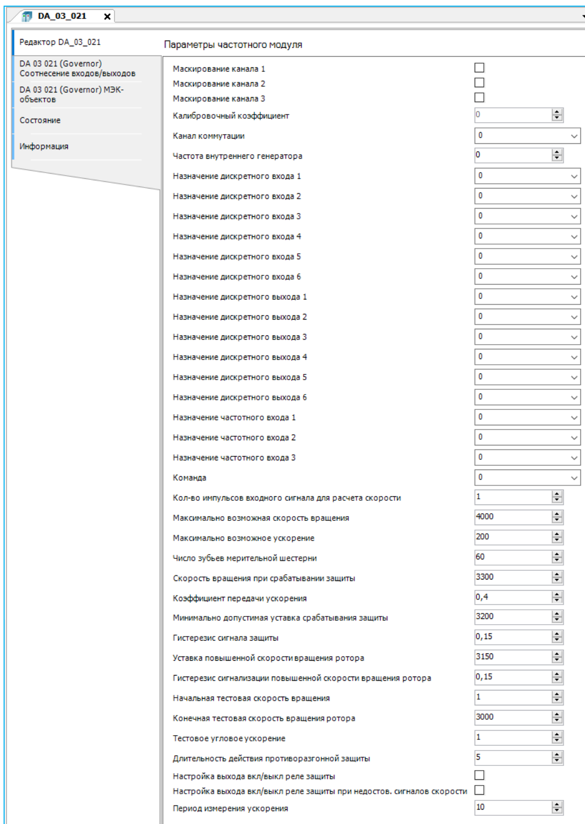
Рисунок 115 – Параметры модуля R600 DA 03 021 (автомат безопасности турбины)
