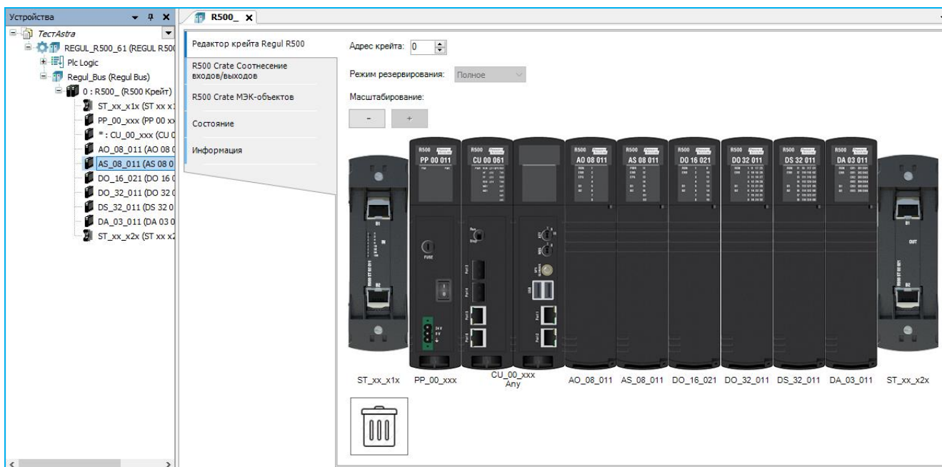
Рисунок 57– Пример редактора крейта (контроллер Regul R500)
