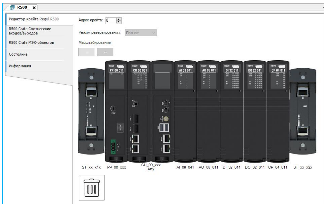
Рисунок 67 – Редактор крейта контроллера Regul R500
