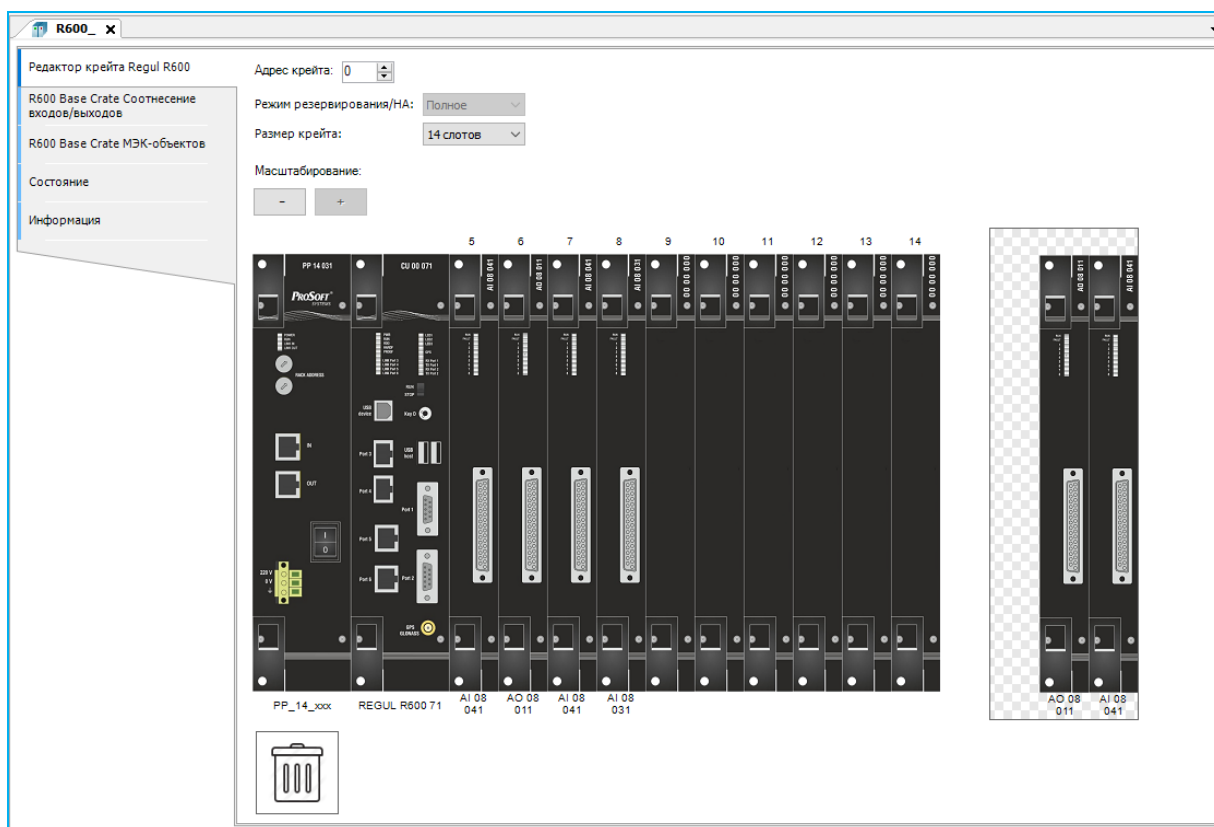
Рисунок 65 – Пример редактора крейта контроллера Regal R600
