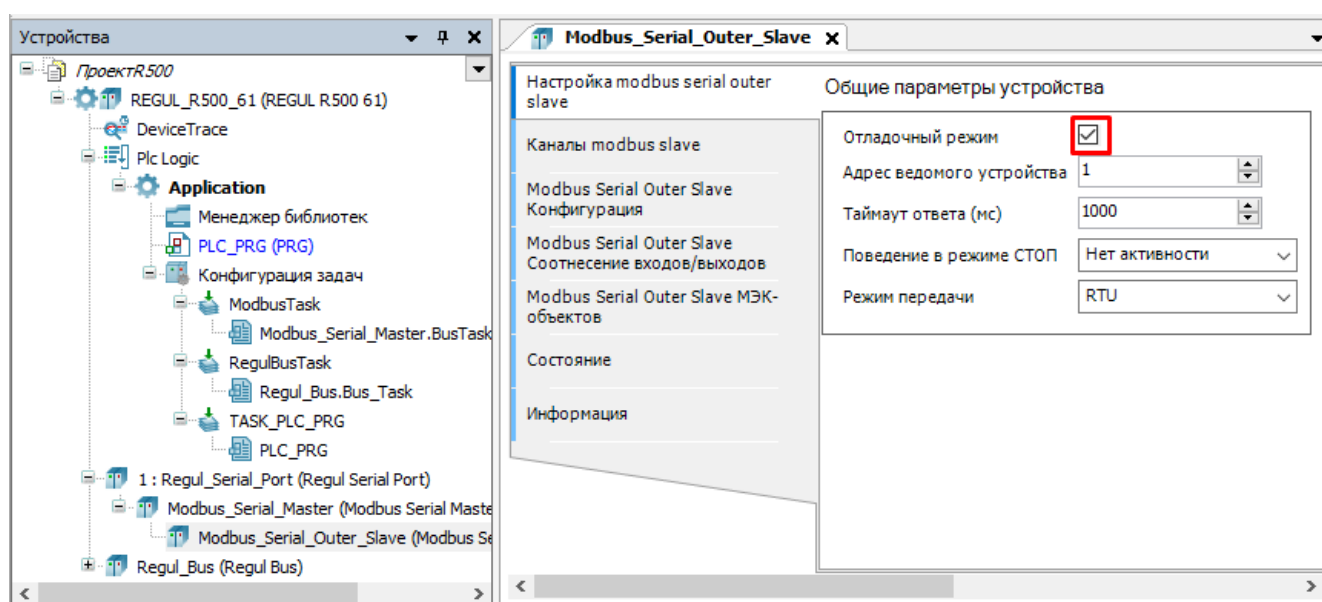
Рисунок 207 – Включение отладочного режима
