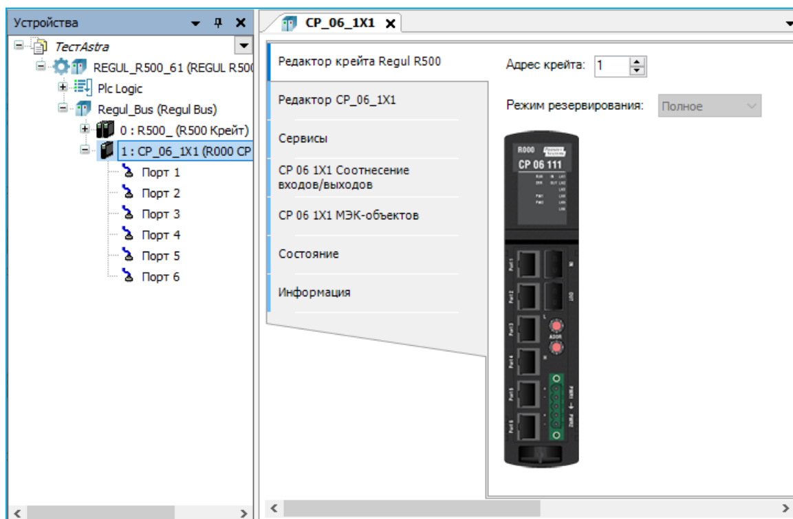
Рисунок 58– Пример редактора Regl R000
