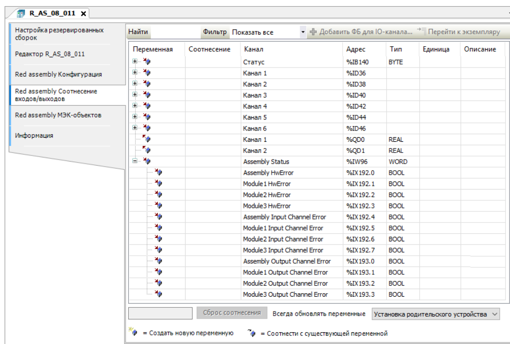
Рисунок 84 – Вкладка соотнесения входов/выходов резервированной сборки на примере модуля R500 AS 08 011
