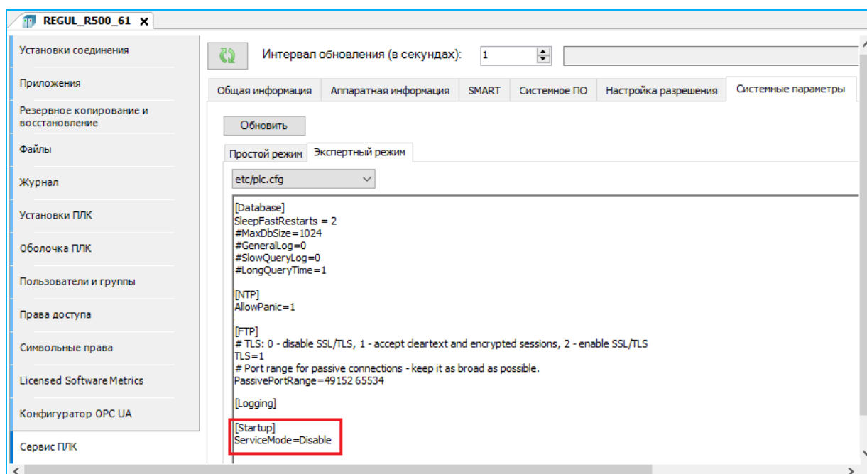
Рисунок 255 – Отключение входа в сервисный режим на время загрузки контроллера
