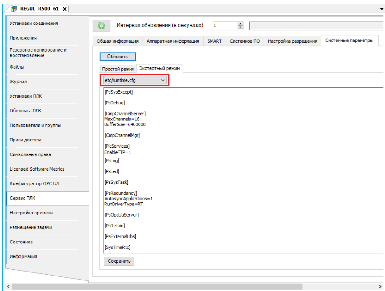
Рисунок 186 – Пример параметров в экспертном режиме для runtime.cfg
