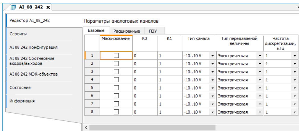
Рисунок 93 – Базовые параметры аналоговых каналов на примере модуля R500 AI 08 242/342
