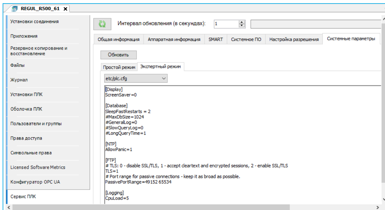
Рисунок 200 – Установка периода журналирования загрузки процессора
