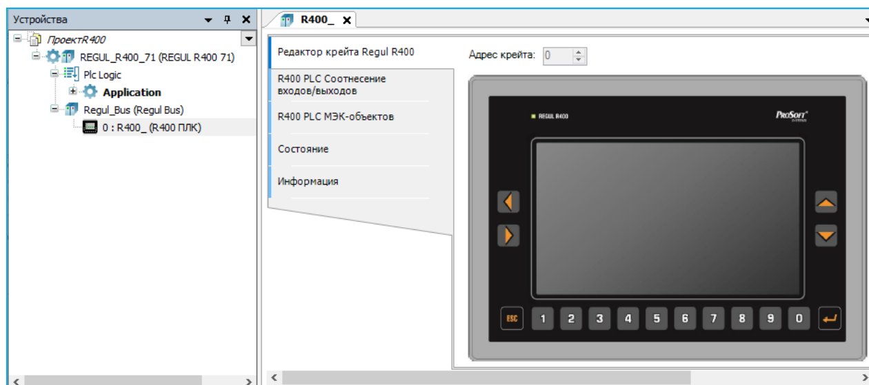
Рисунок 74 – Редактор крейта контроллера Regul R400
