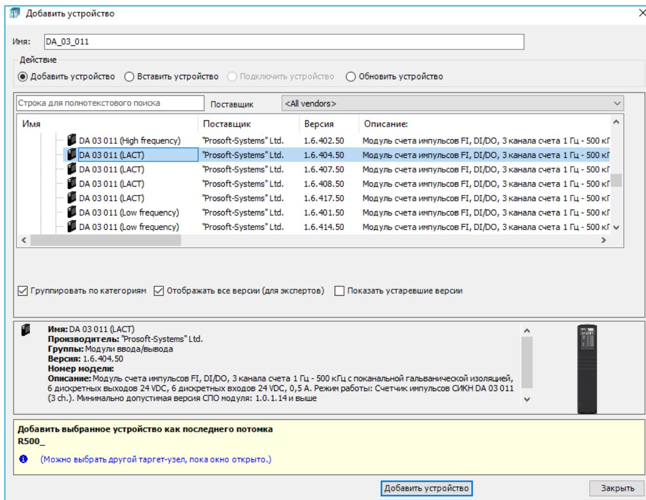
Рисунок 64 – Список модулей всех версий
