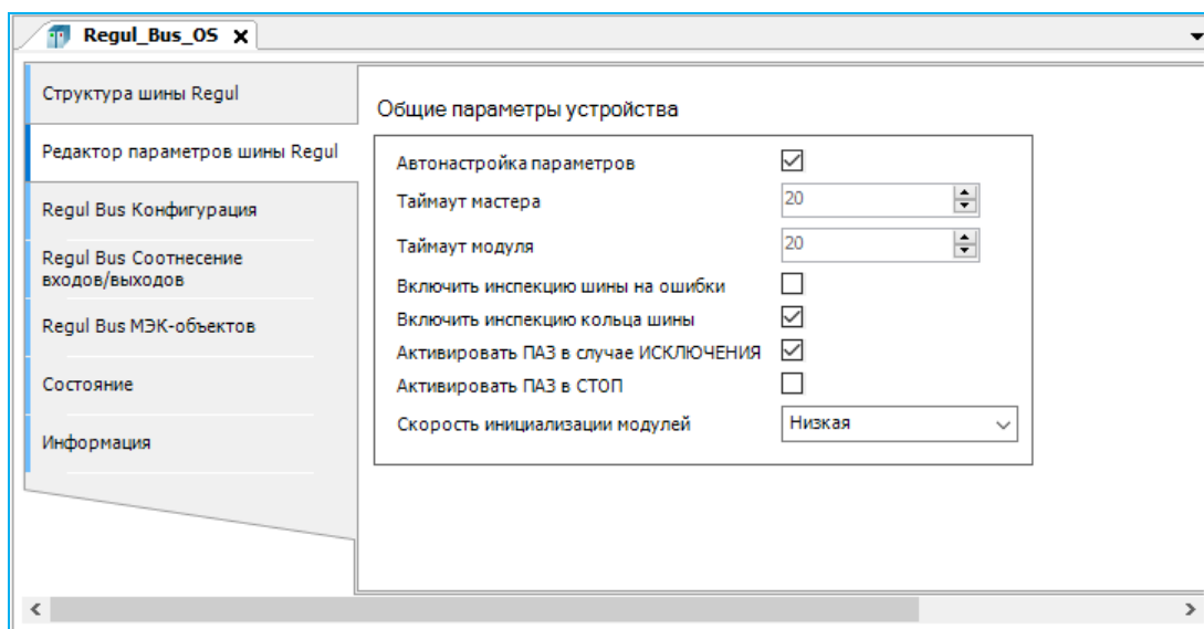
Рисунок 55 – Редактор параметров шины RegulBus OS (для III-го типа модулей)
