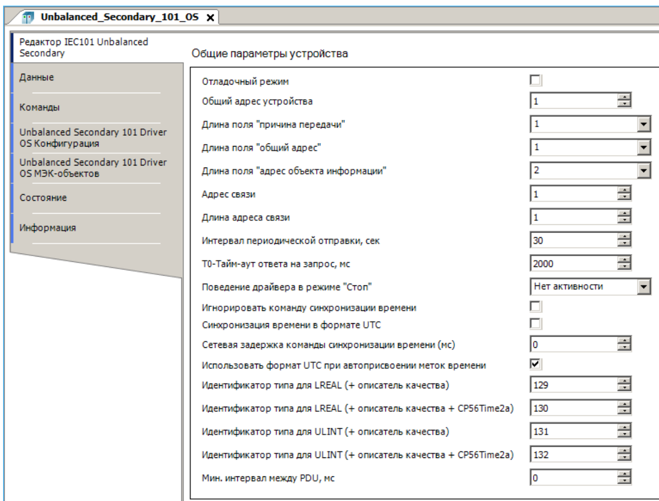
Рисунок 63 - Редактор устройства IEC101 Unbalanced Secondary
