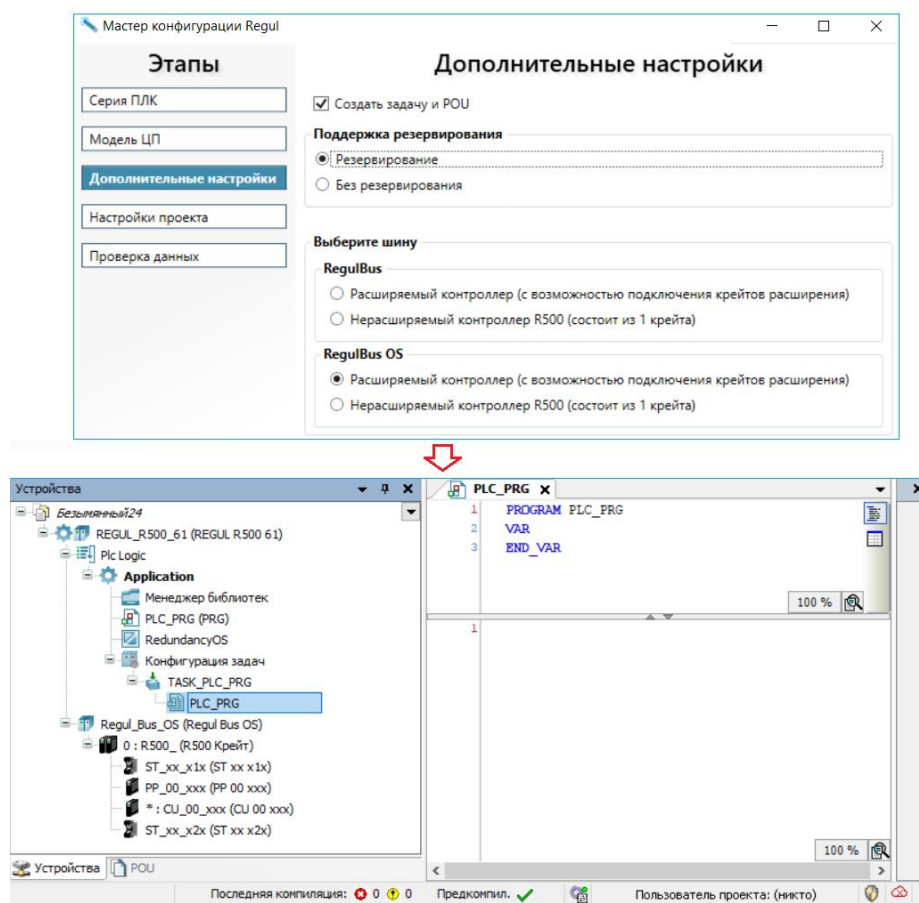
Рисунок 24 – Автоматическое добавление компонента «Резервирование» при создании нового проекта начиная с версии 1.7.1.0
