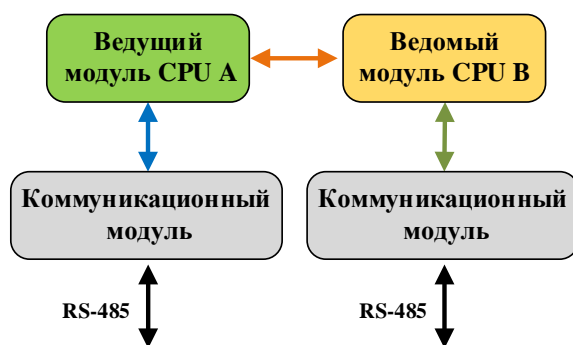
Рисунок 36 – Трансляция данных с модулей ЦП в схеме полного резервирования через коммуникационные модули RS-485
