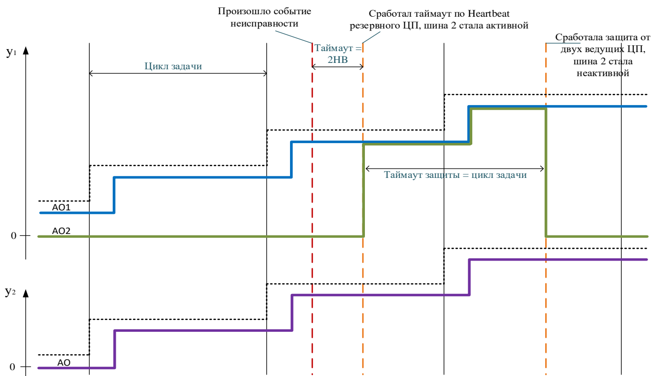
Рисунок 22 – Поведение сигнала при аппаратной неисправности линии связи между модулями ЦП
