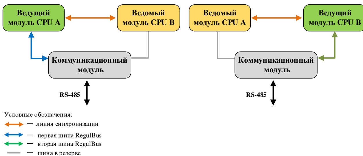
Рисунок 35 – Трансляция данных с модулей ЦП в схеме частичного резервирования через коммуникационные модули RS-485
