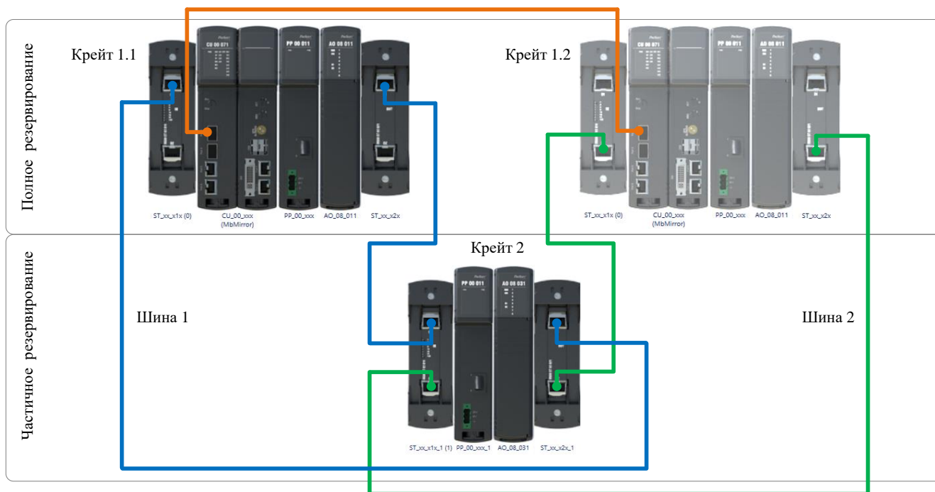
Рисунок 18 – Комбинированная схема резервирования
