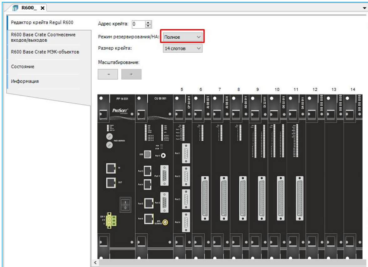
Рисунок 25 – Пример редактора крейта (контроллер ReguL R600)
