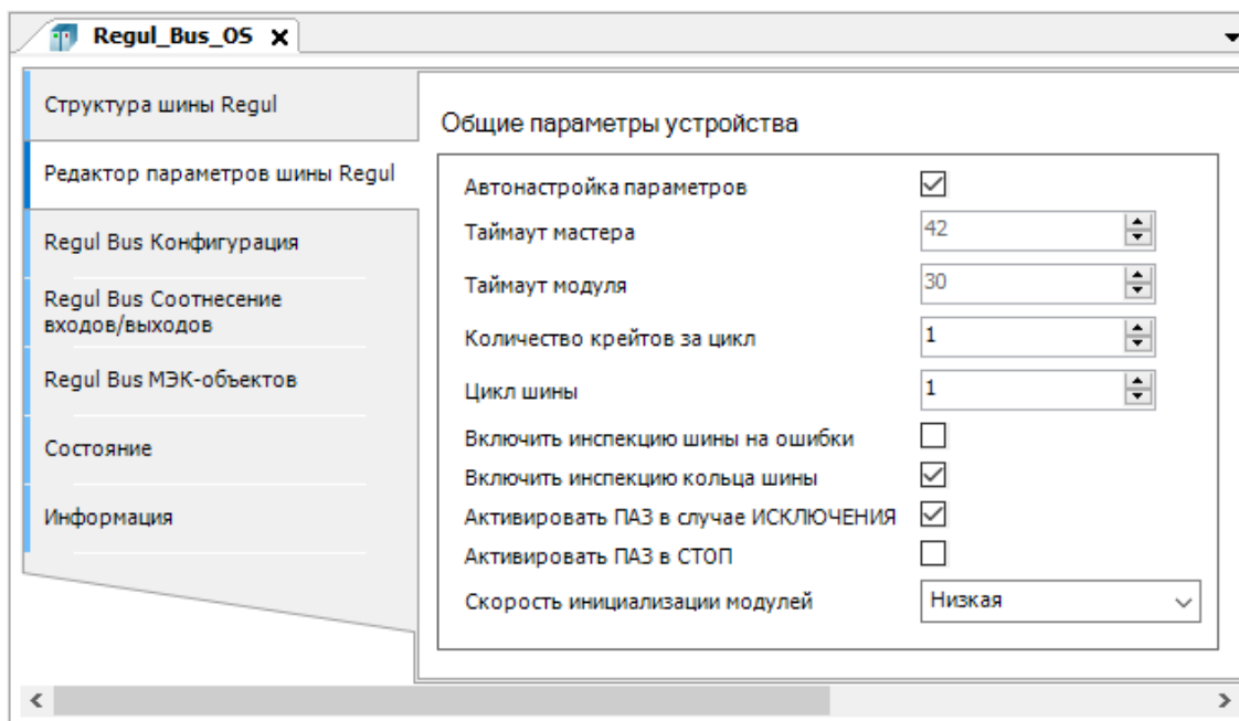
Рисунок 16 - Редактор параметров шины RegulBus OS
