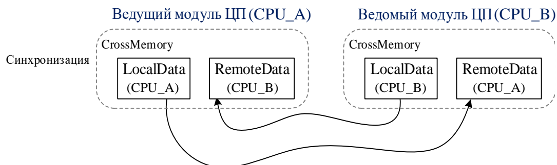
Рисунок 39 – Блок CrossMemory
