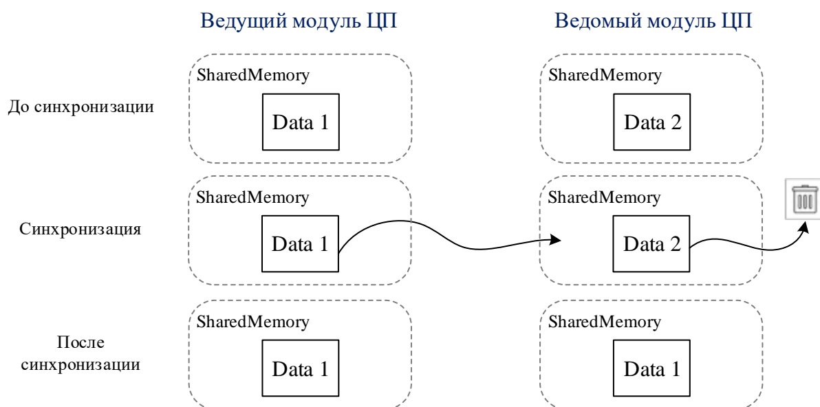
Рисунок 38 – Блок SharedMemory
