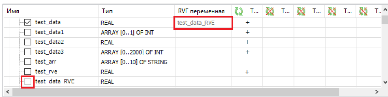
Рисунок 53
