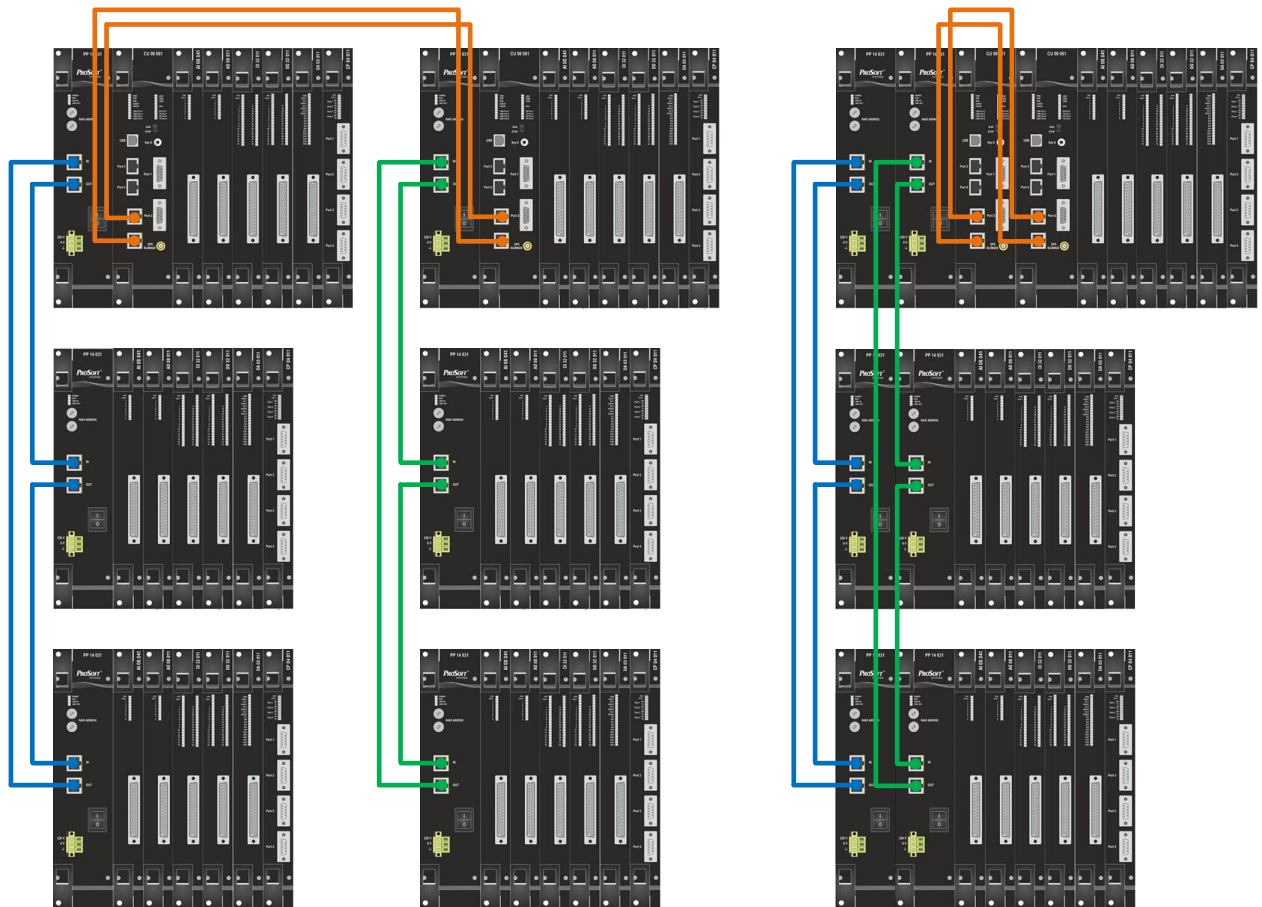
Рисунок 6 – Примеры схем полного и частичного резервирования, Regul R600
