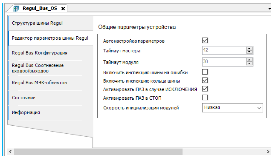
Рисунок 17 – Редактор параметров шины RegulBus OS (для III-го типа модулей)
