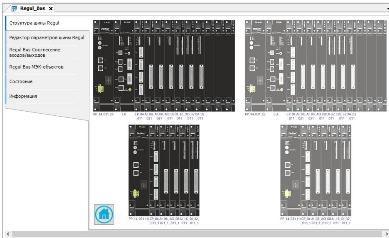
Рисунок 27 – Редактор шины контроллера R600 (2 крейта, с полным резервированием)
