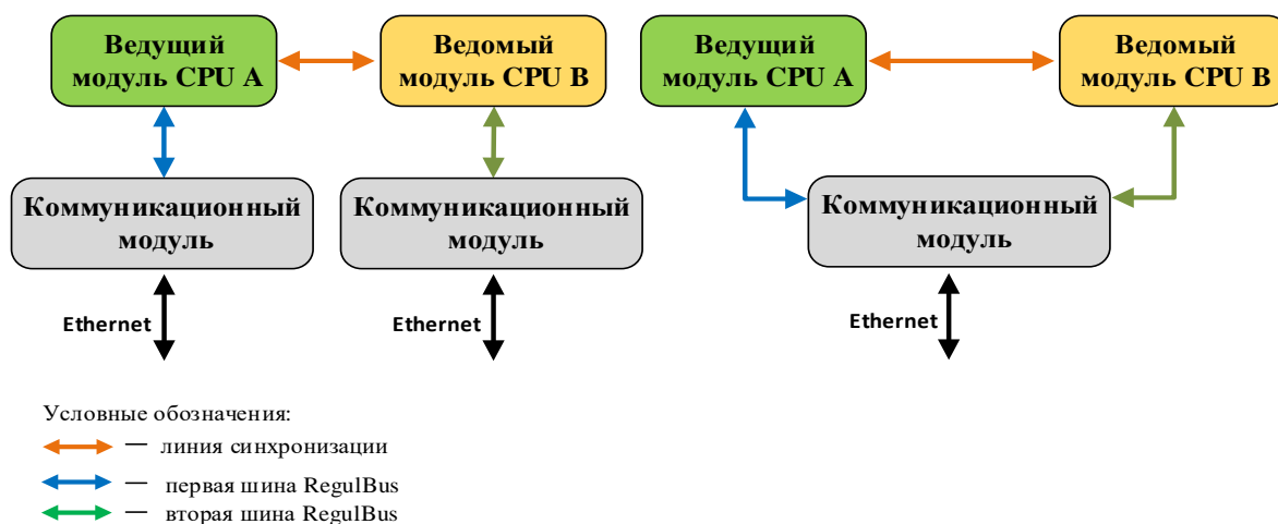
Рисунок 33 – Трансляция данных с модулей ЦП в различных схемах резервирования
