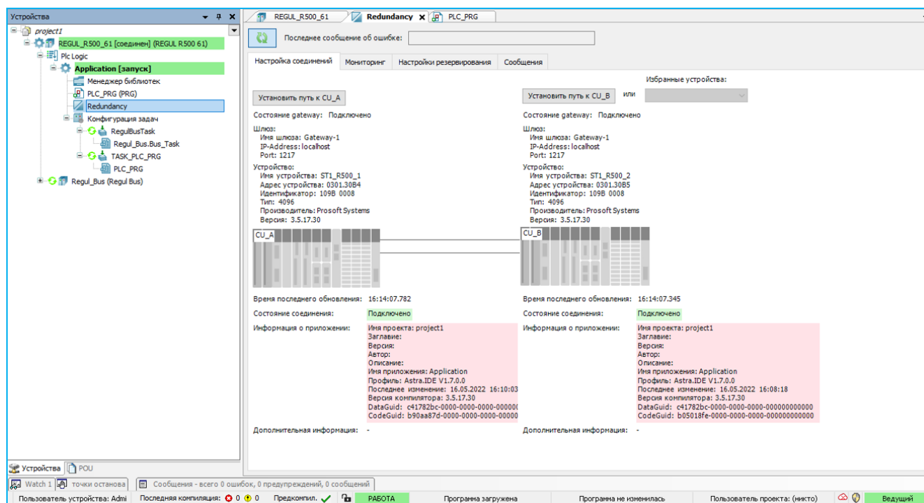
Рисунок 67 – Вкладка «Настройка соединений». Резервный контроллер находится в состоянии Standby, что сигнализирует о синхронизации данных проекта, но загружены разные проекты на модулях ЦП (информация о приложениях помещена на красном фоне)
