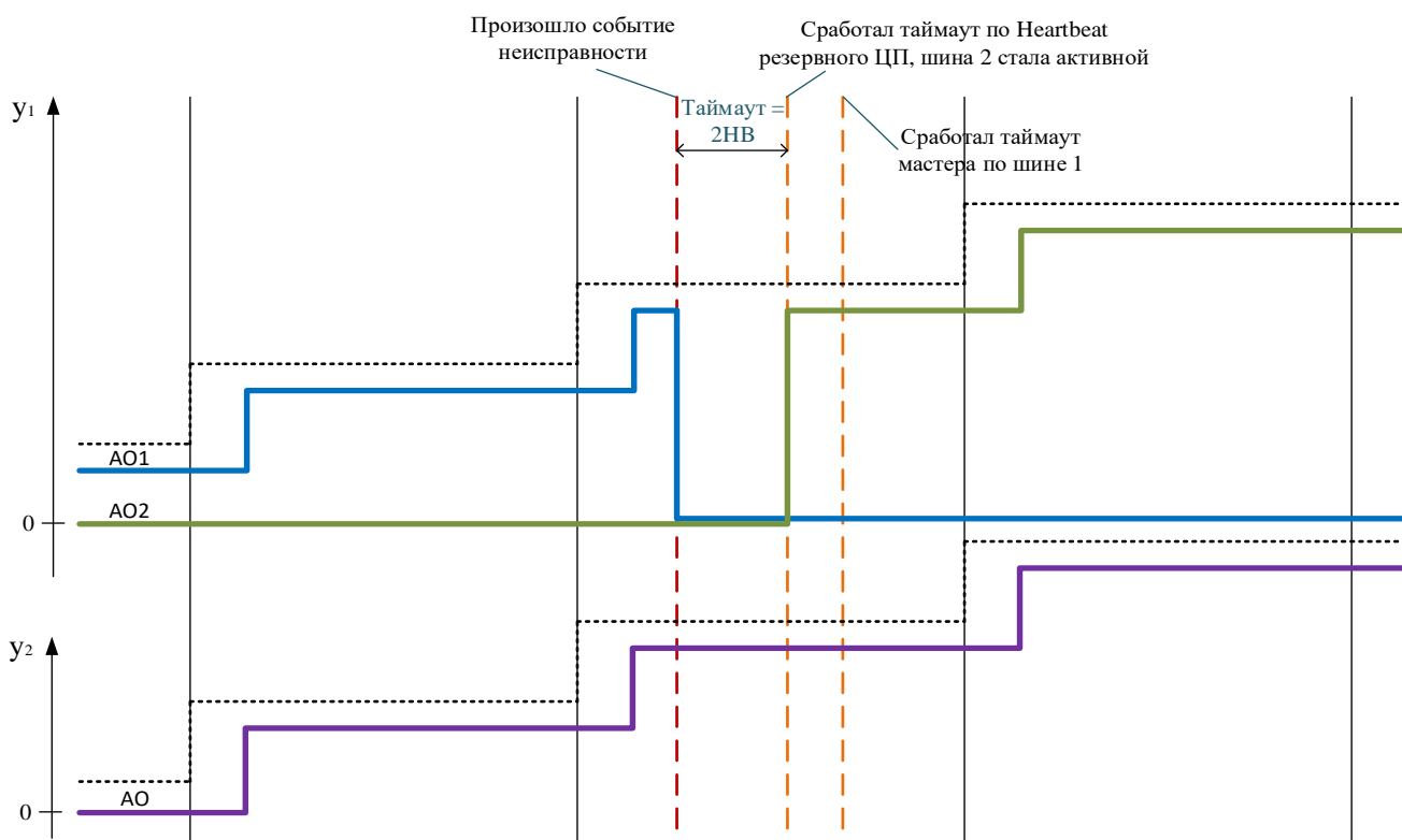
Рисунок 20 – Поведение сигнала при отсутствии питания в крейте 1.1
