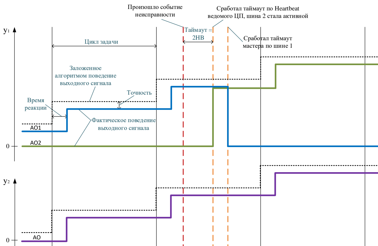
Рисунок 19 – Поведение сигнала при выходе из строя модуля ЦП1
