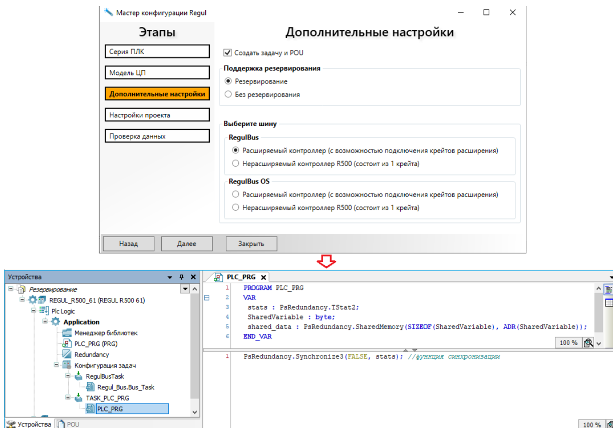
Рисунок 23 – Автоматическое добавление компонента «Резервирование» при создании нового проекта до версии 1.7.1.0
