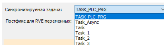
Рисунок 44 – Синхронизируемая задача
