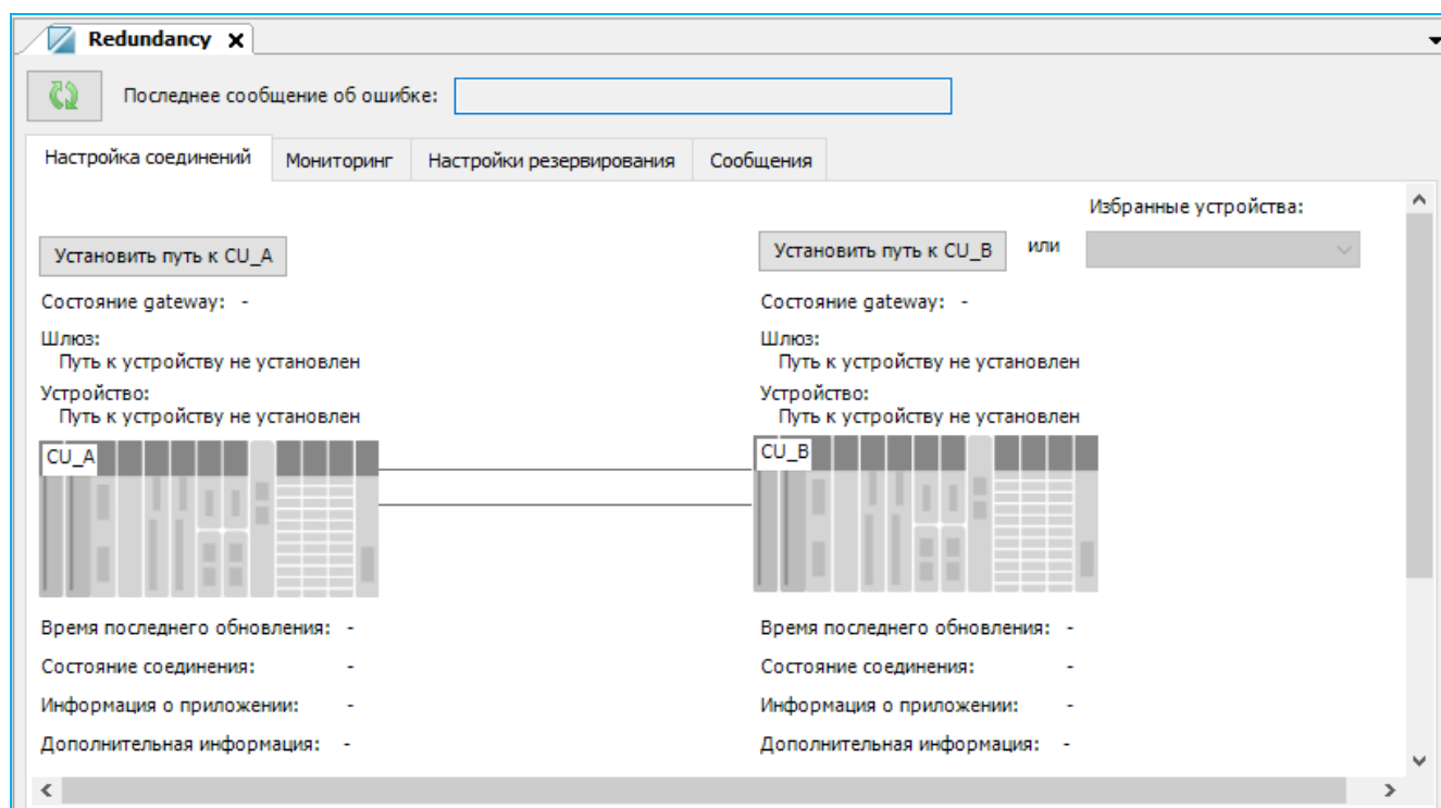
Рисунок 55 – Резервирование. Настройка соединений
