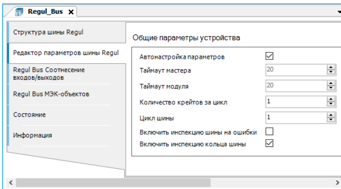
Рисунок 15 - Редактор параметров шины RegulBus
