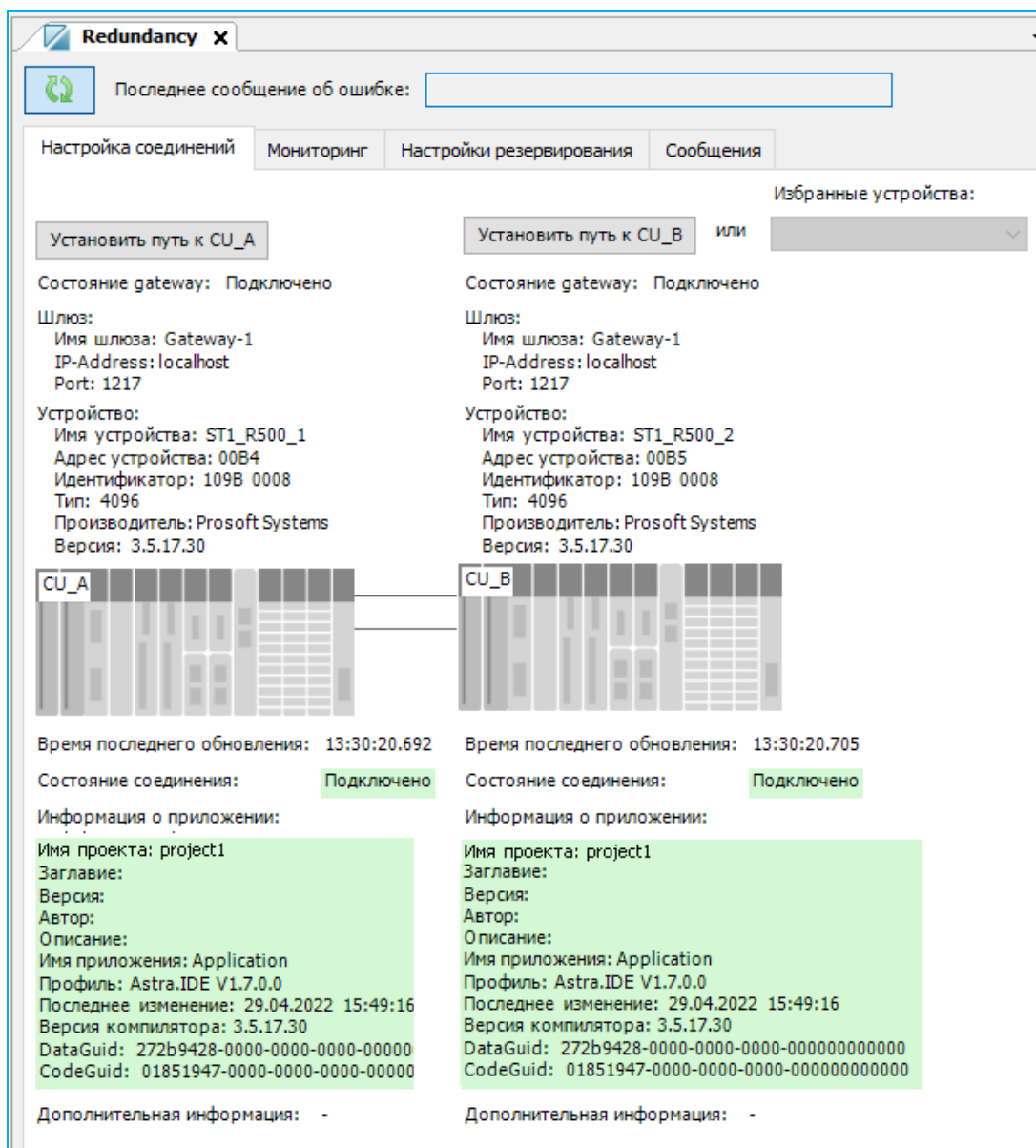
Рисунок 57 – Резервирование. Настройка соединений и текущее состояние модулей ЦП
