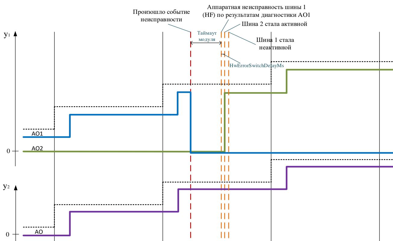
Рисунок 21 – Поведение сигнала при аппаратной неисправности модуля AO1 в крейте 1.1
