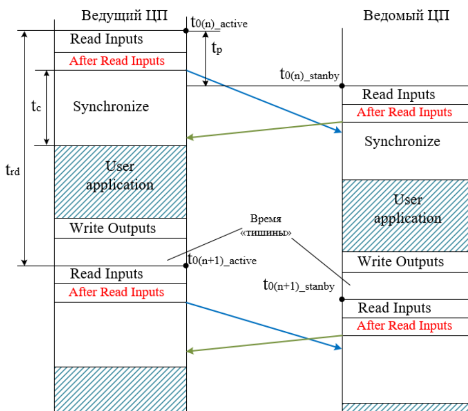
Рисунок 41 – Алгоритм работы задачи резервирования с AfterReadingInputs
