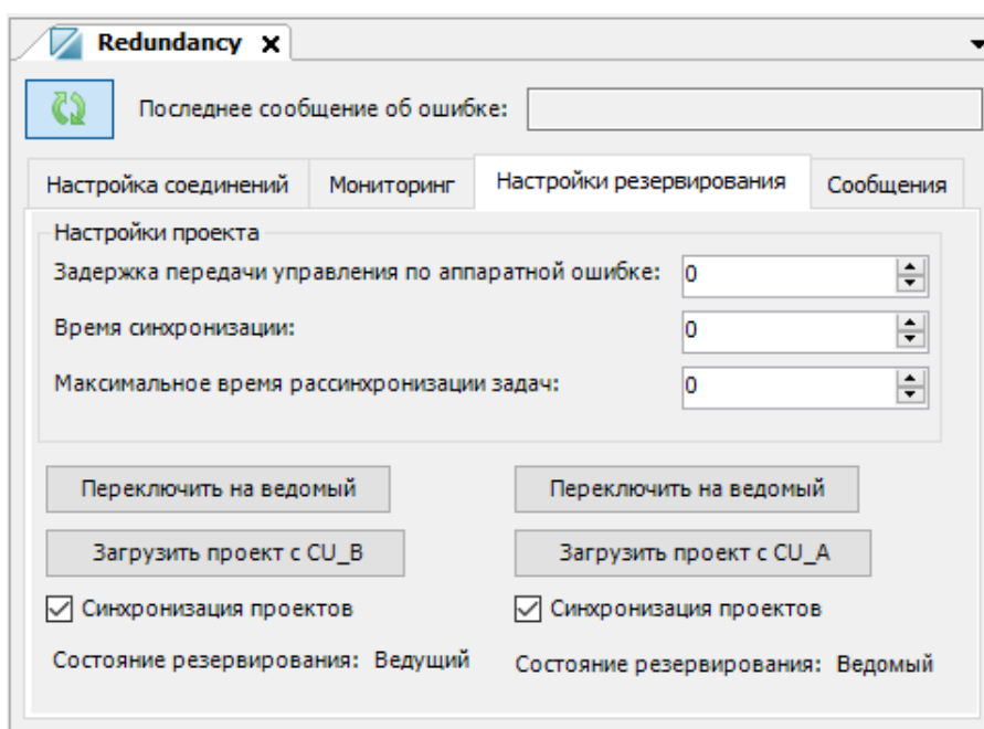
Рисунок 59 – Настройка параметров модулей ЦП (CU_A/B)
