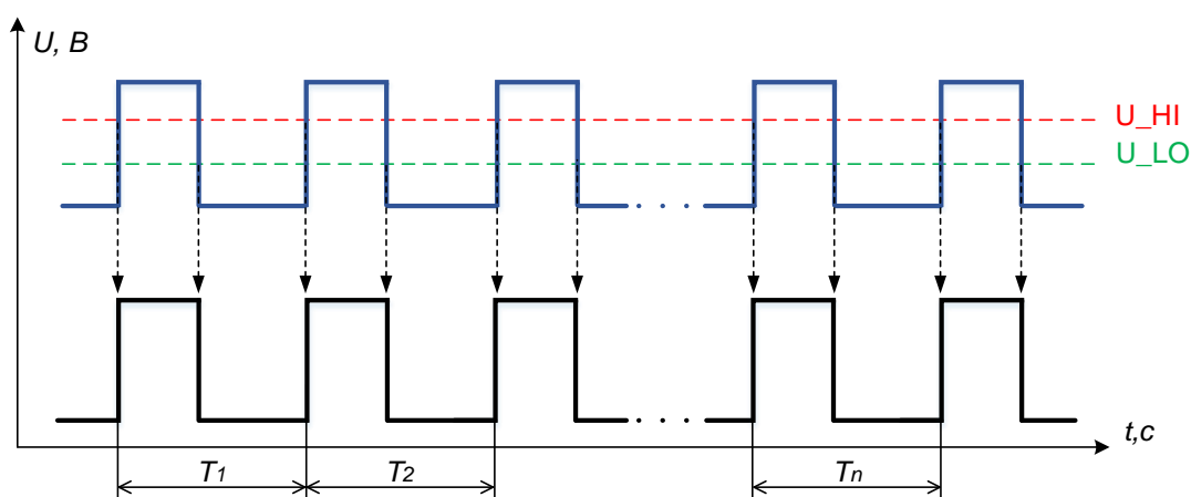
Рисунок 75 – Детектирование сигнала
