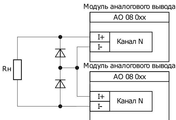
Рисунок В.9 – Подключение не резервированного аналогового исполнительного устройства к резервированным каналам вывода аналоговых сигналов.
