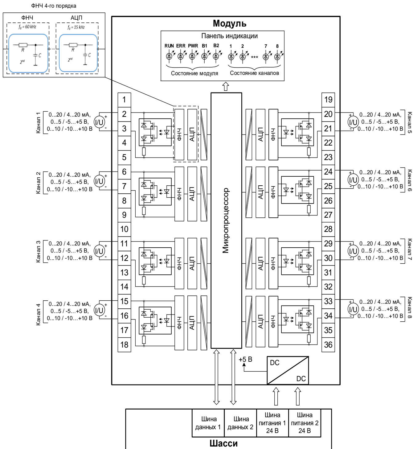
Рисунок 53- Структурная схема модуля AI 08 242
