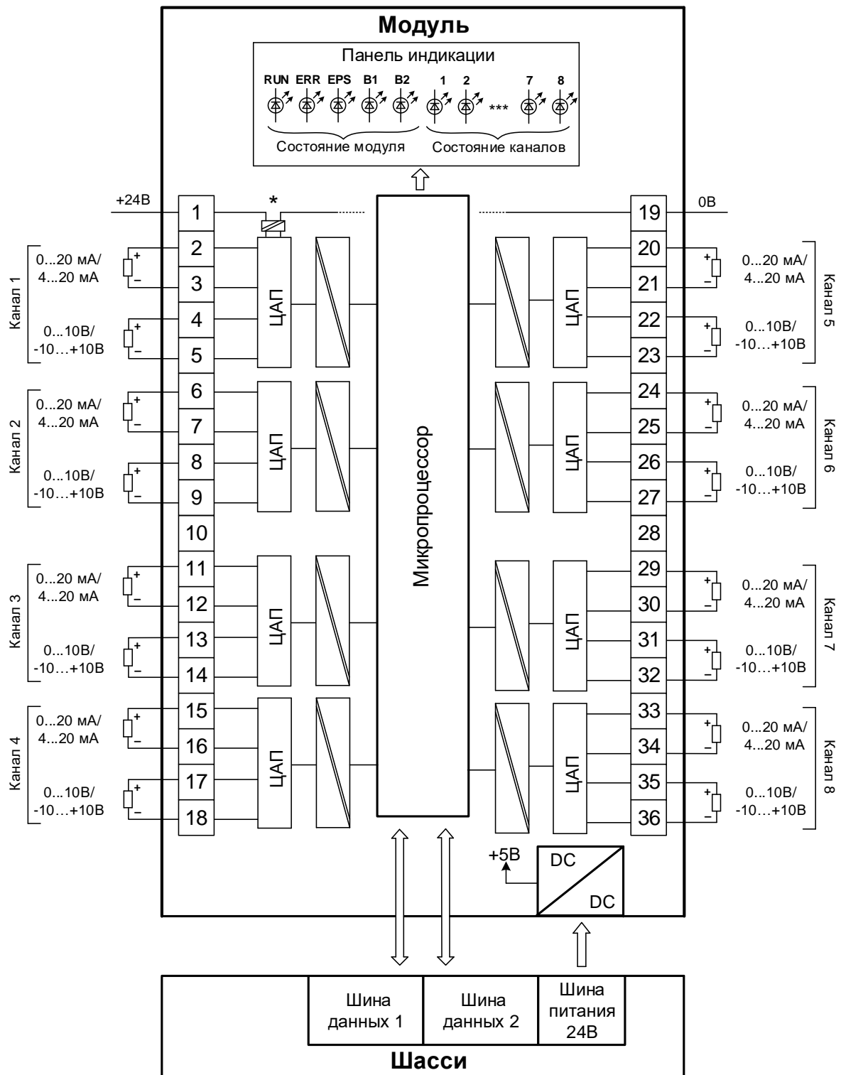
Рисунок 61 - Структурная схема модуля АО 08 031
