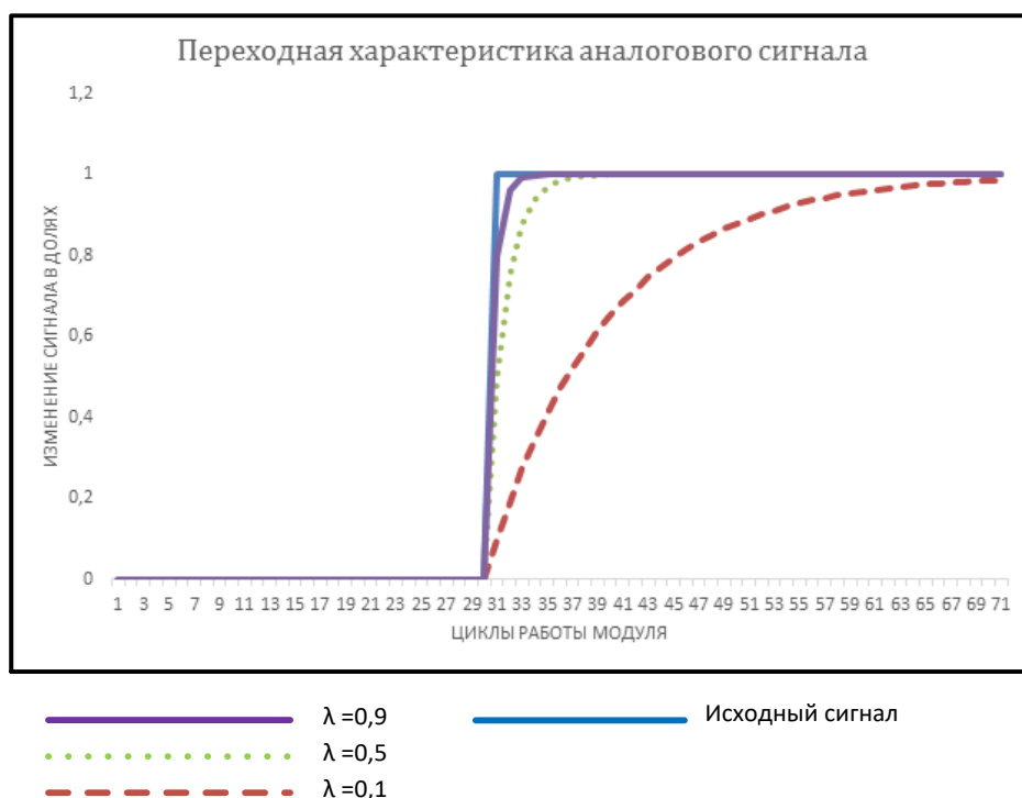
Рисунок 46 - Зависимость аналогового сигнала от коэффициента усреднения \lambda
