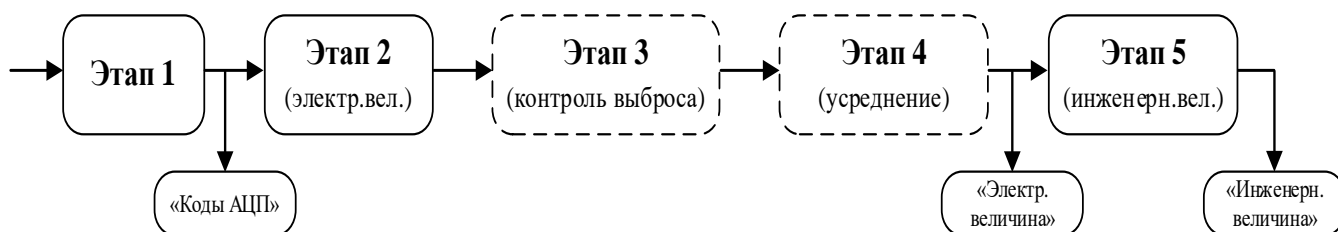
Рисунок 43 - Этапы преобразования сигнала
