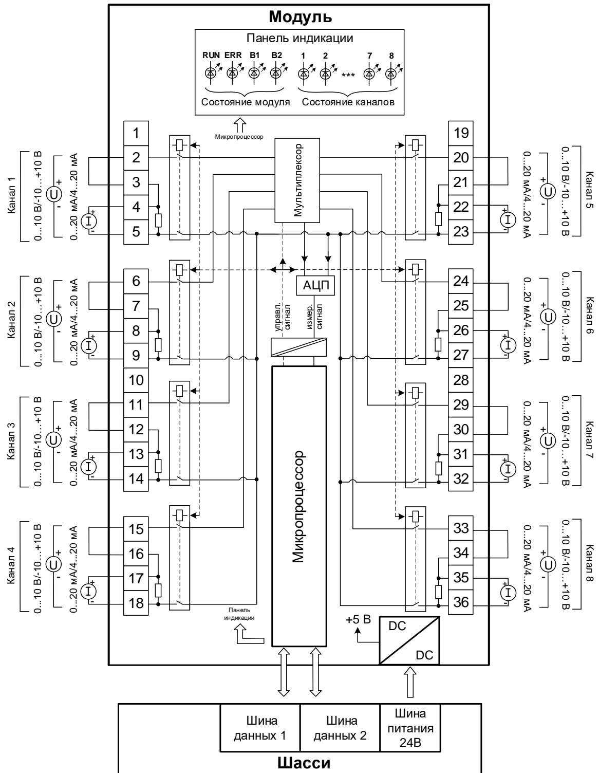
Рисунок 55 – Структурная схема модуля AI 08 051
