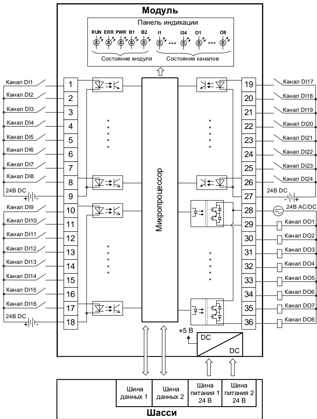
Рисунок 74 - Структурная схема модуля DS 32 012
