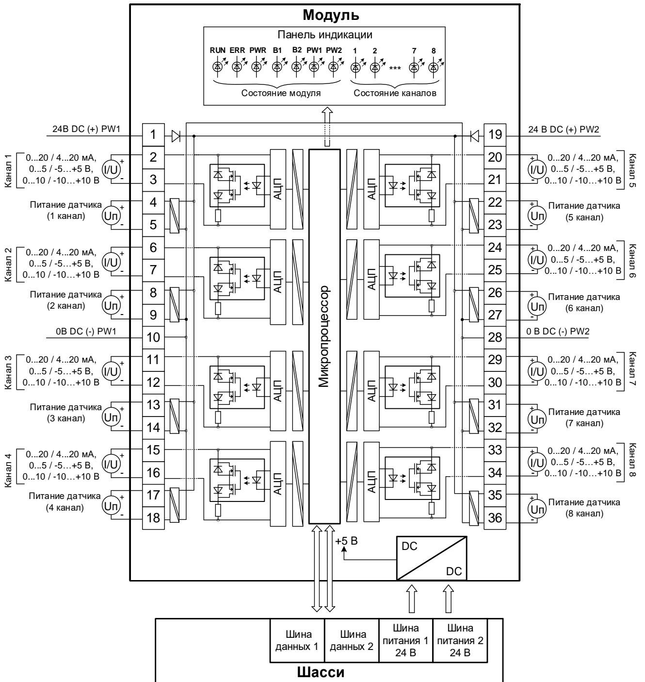
Рисунок 52 - Структурная схема модуля AI 08 142
