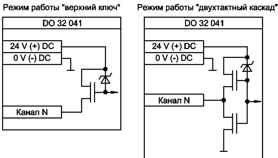
Рисунок 70 – Структурные схемы модуля одного из каналов в различных режимах работы
