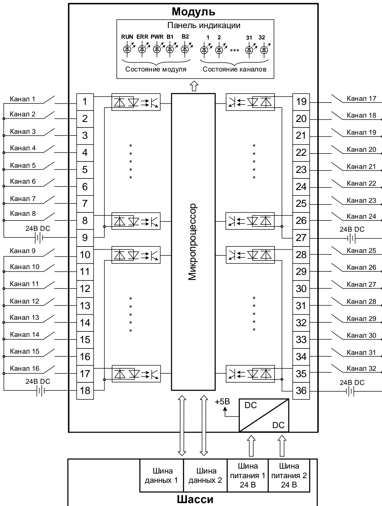
Рисунок 64 - Структурная схема модуля DI 32 012, DI 32 013
