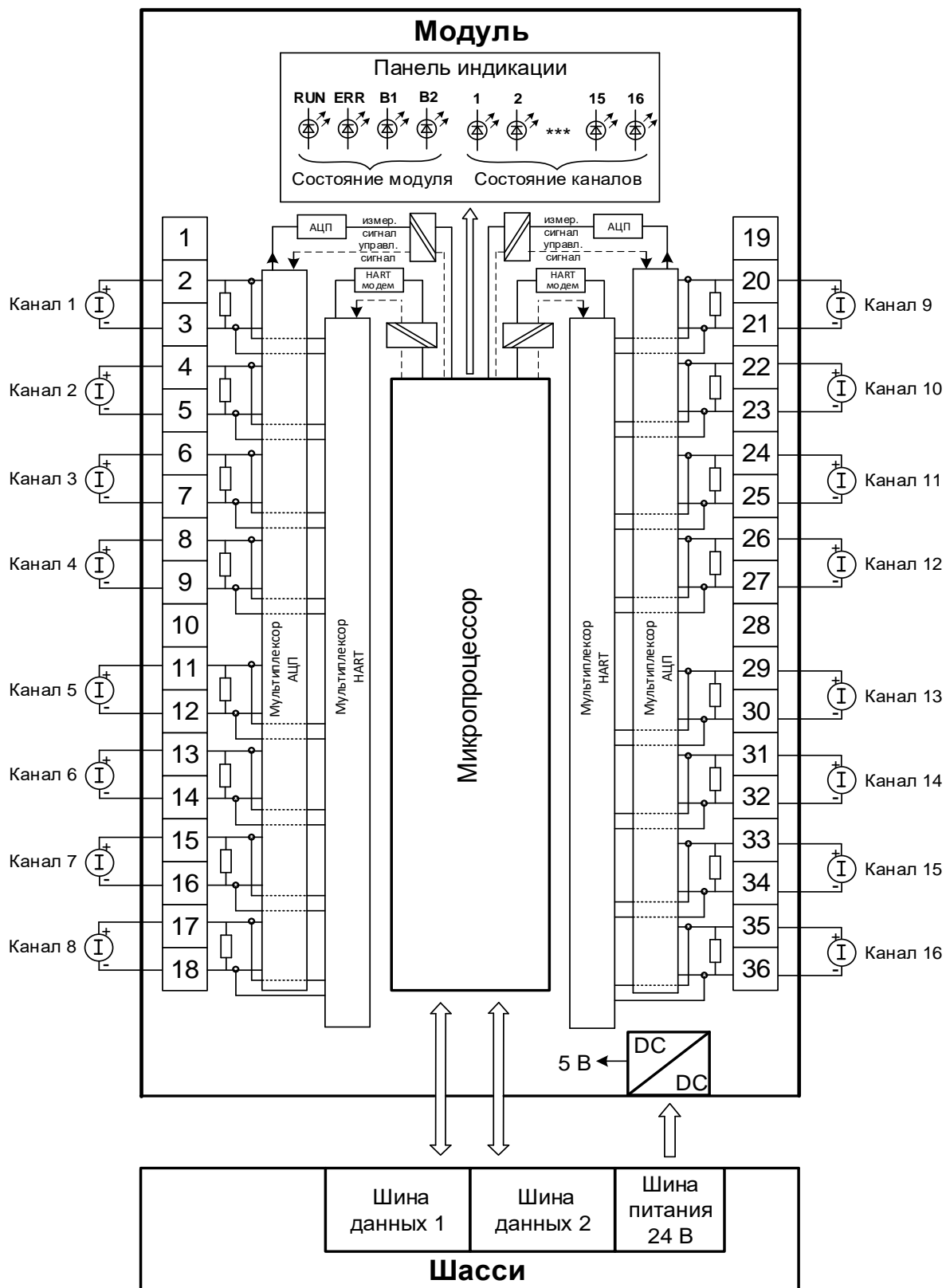
Рисунок 58 - Структурная схема модуля AI 16 081
