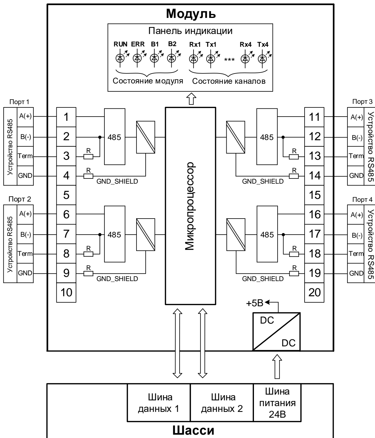
Рисунок 39 - Структурная схема модуля CP 04 011
