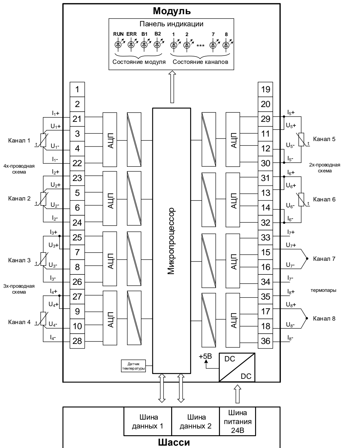
Рисунок 48 - Структурная схема модуля AI 08 131
