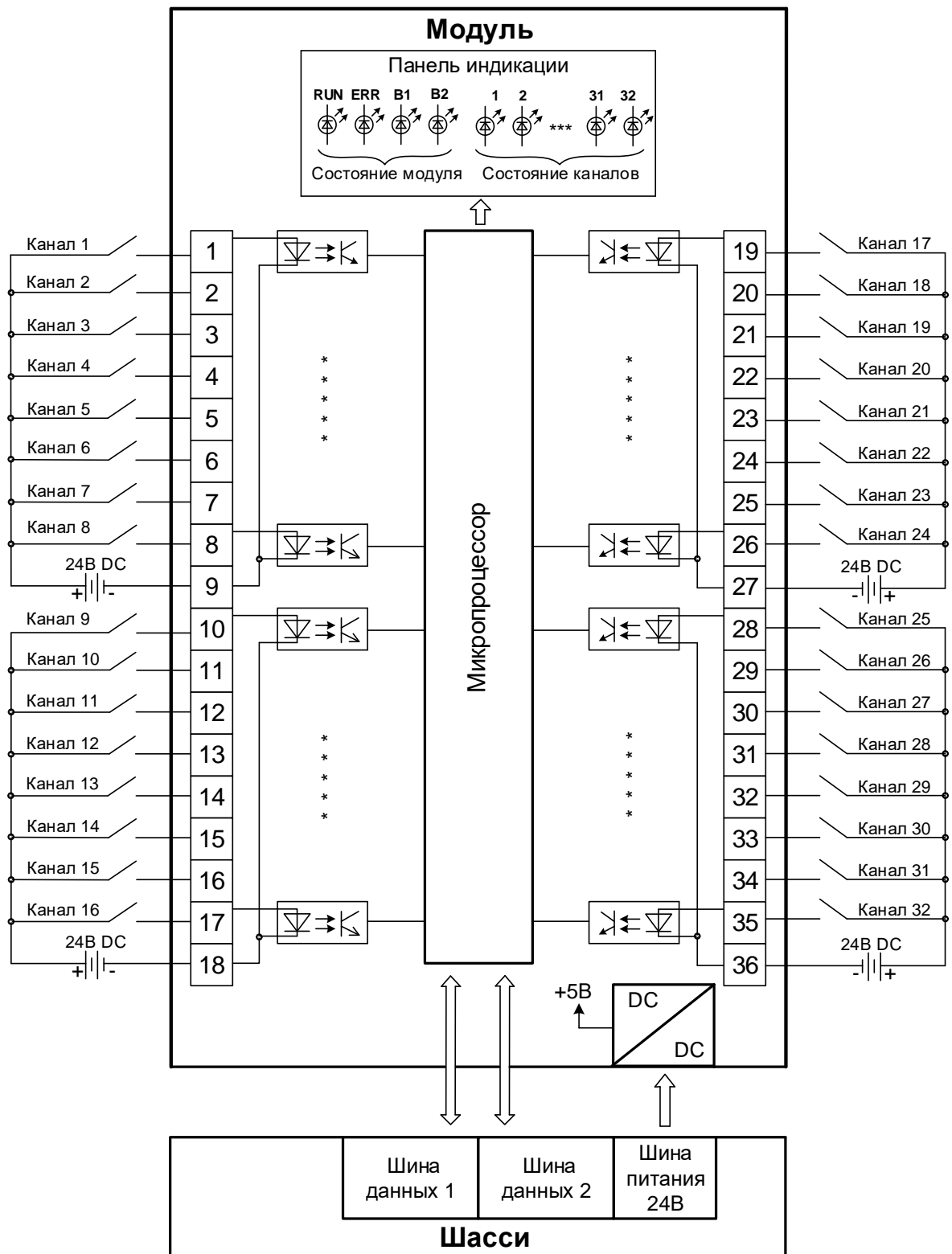
Рисунок 63 - Структурная схема модуля DI 32 011
