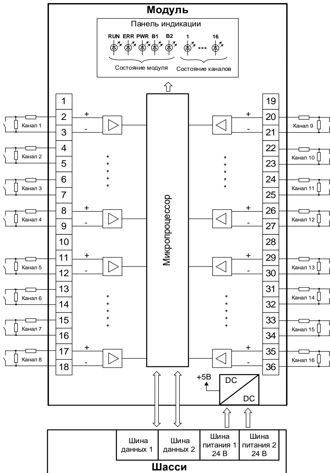
Рисунок 67 – Структурная схема модуля DI 16 032
