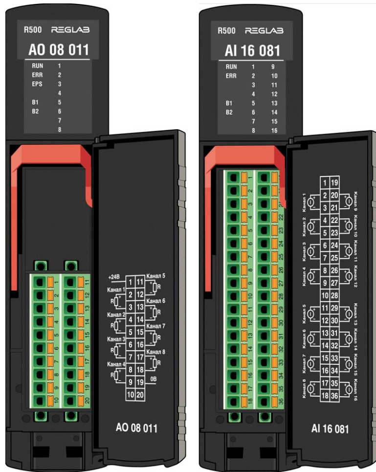
Рисунок 83- Модули аналогового ввода АО 08 011 и АІ 16 081 с клеммными колодками, на 20 и 36 контактов соответственно
