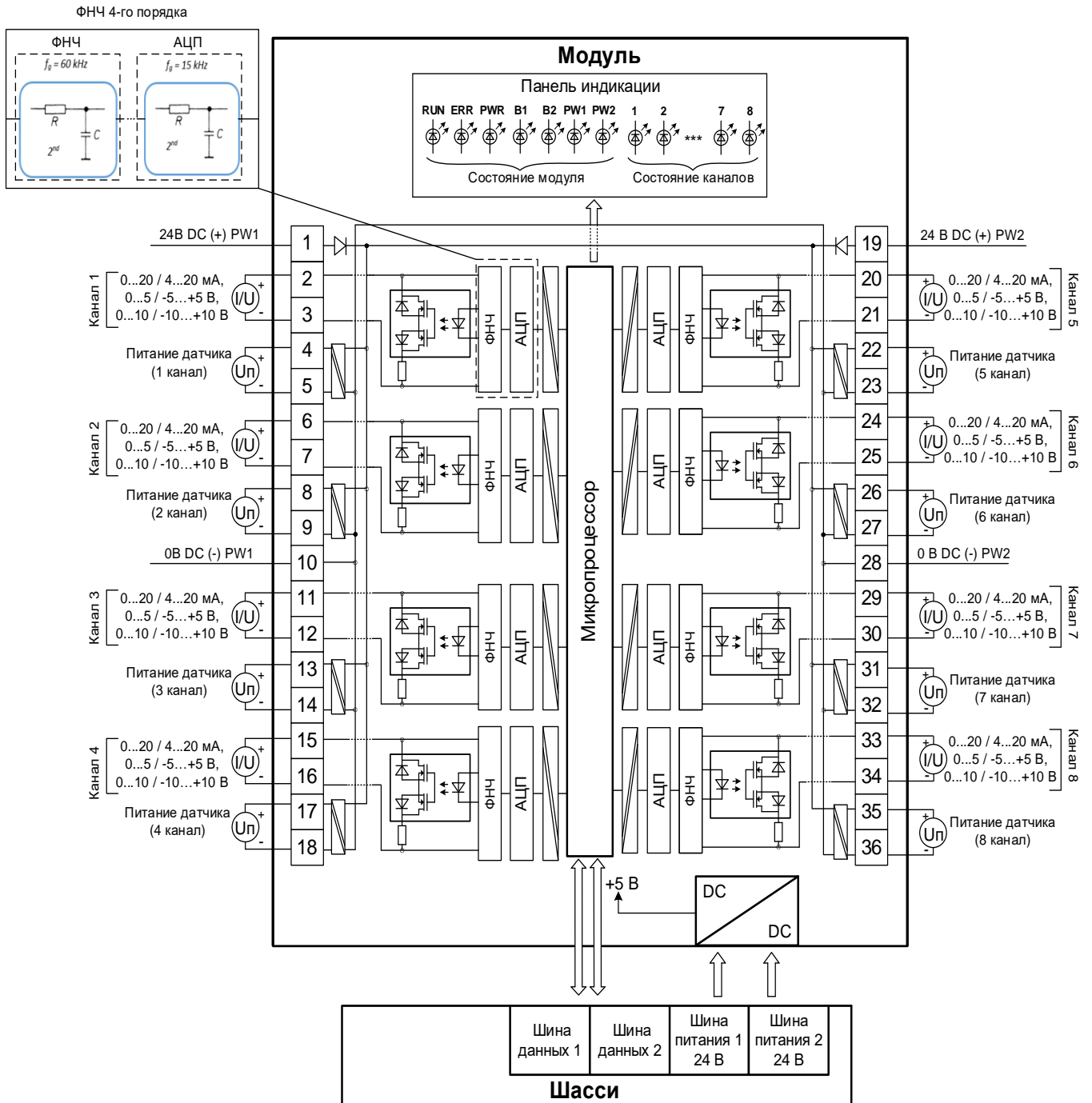
Рисунок 54- Структурная схема модуля AI 08 342
