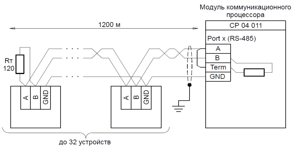
Рисунок Б.6.4 – Схема подключения устройств к модулям коммуникационного процессора
