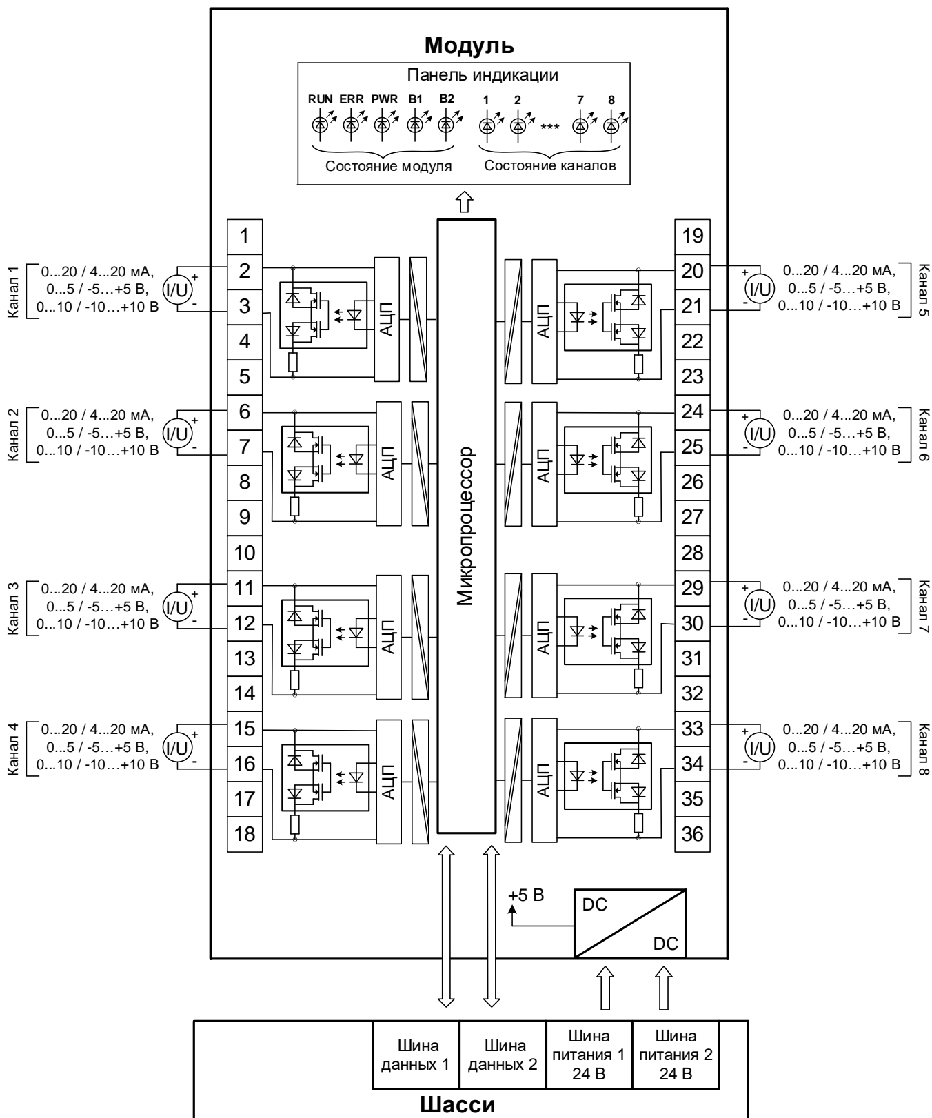
Рисунок 50 – Структурная схема модуля AI 08 042
