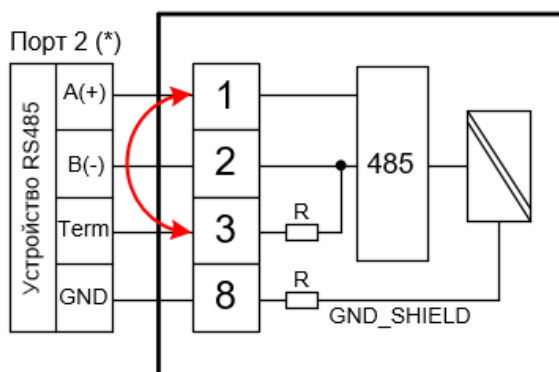
Рисунок 37 – Установка перемычки
