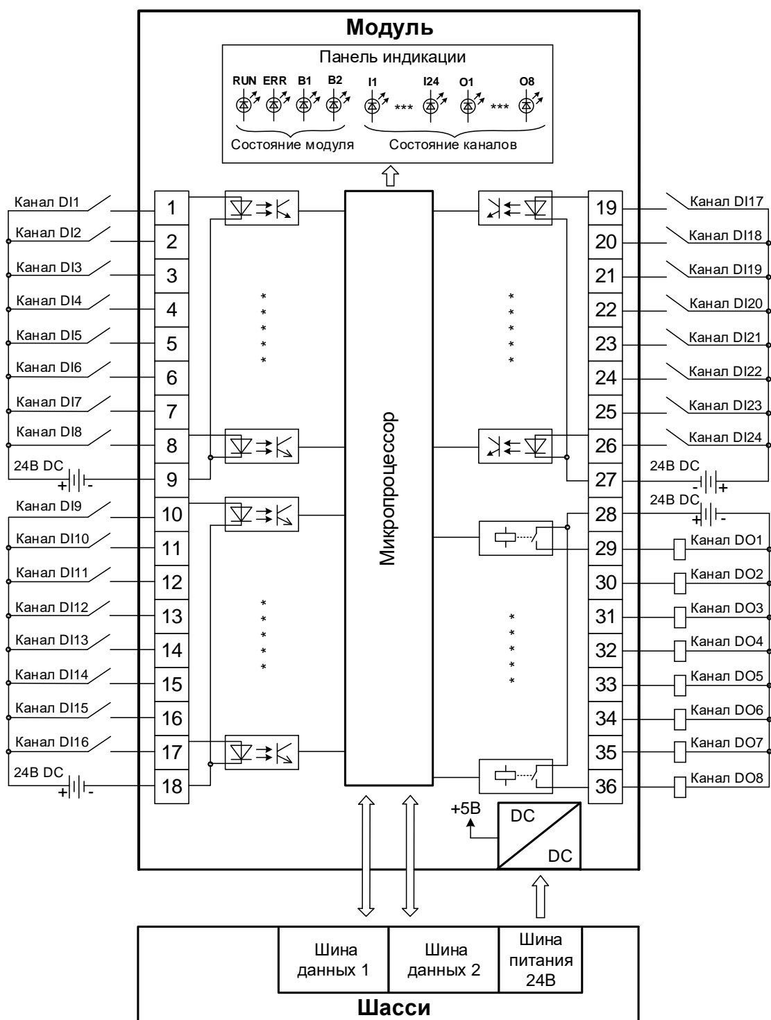
Рисунок 73 - Структурная схема модуля DS 32 011
