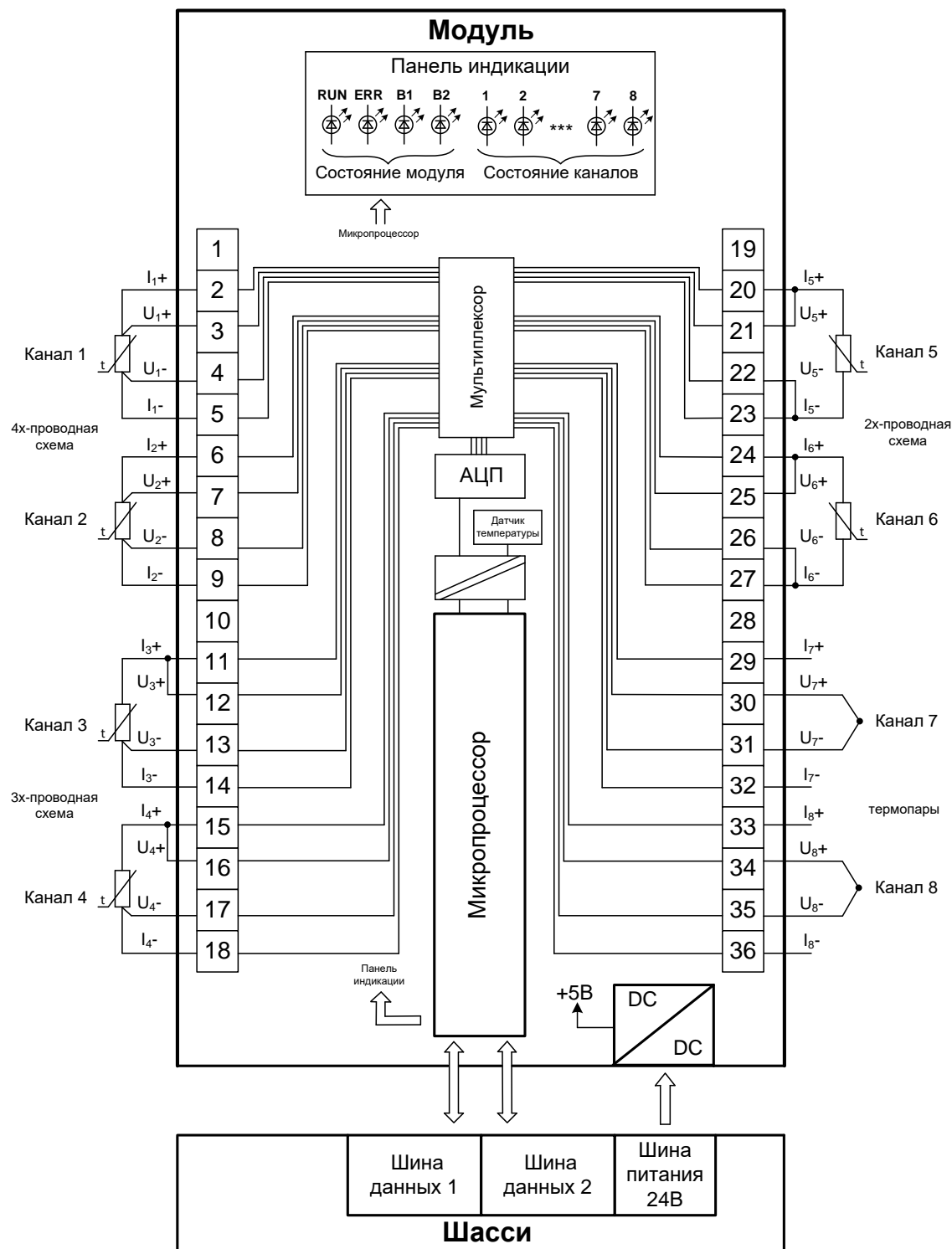
Рисунок 47 - Структурная схема модуля AI 08 031
