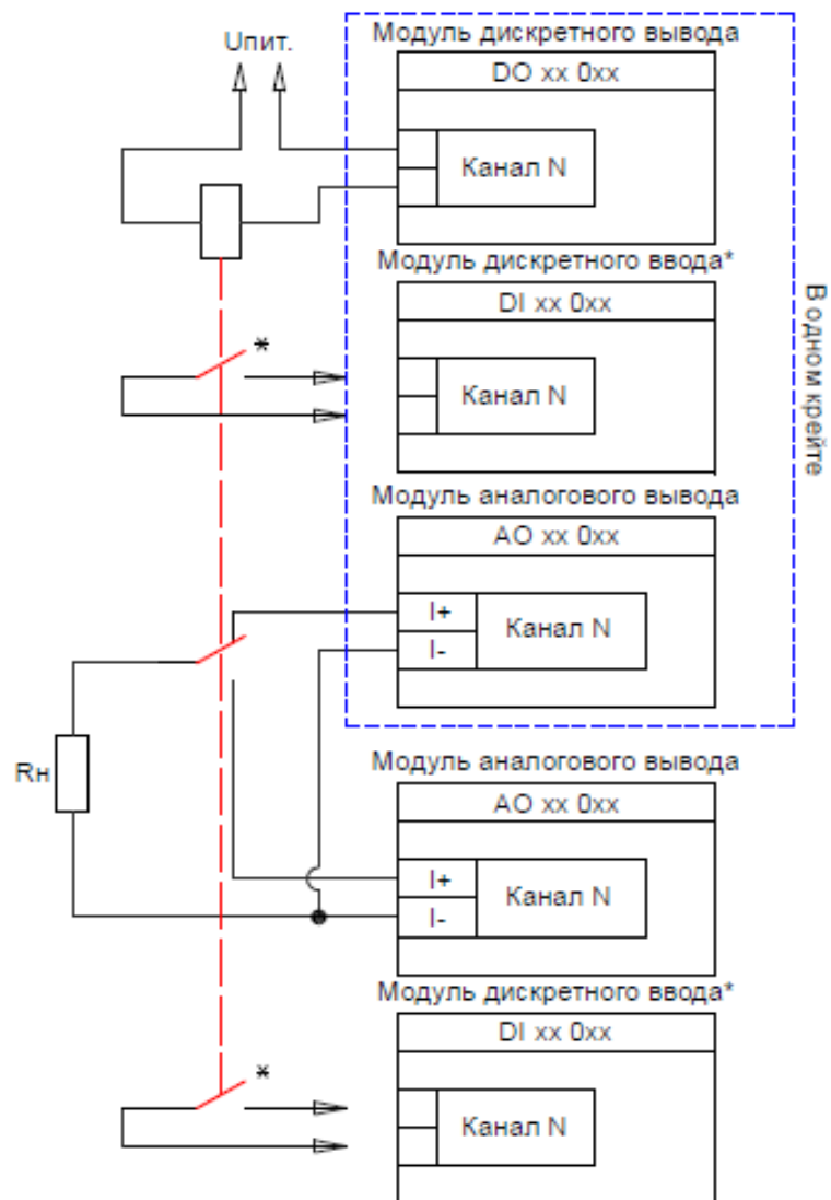
Рисунок В.6 – Подключение не резервированного аналогового исполнительного устройства к резервированным каналам вывода аналоговых сигналов
