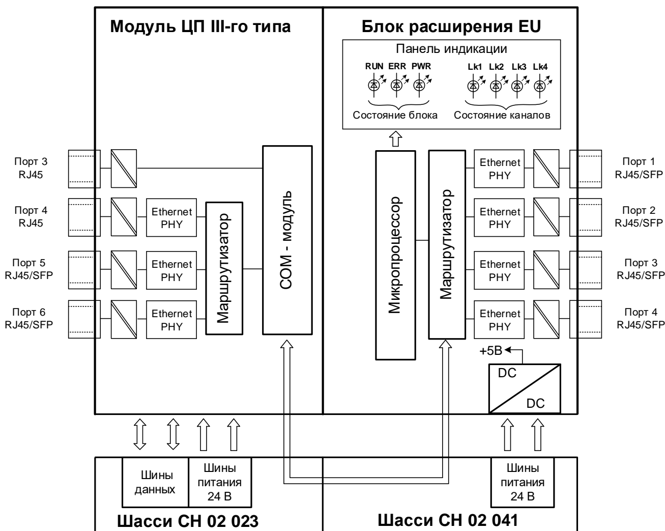
Рисунок 38 - Структурная схема блока расширения EU (для EU 04 021 – порты RJ45, для EU 04 031 - порты SFP)
