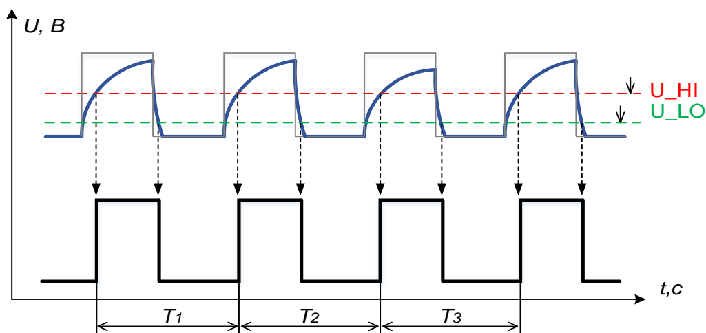
Рисунок 77 – Оптимальные условия детектирования сигнала на высоких частотах
