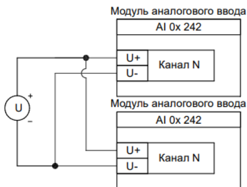
Рисунок В.7 - Подключение не резервированного датчика напряжения к резервированным каналам ввода аналоговых сигналов напряжения
