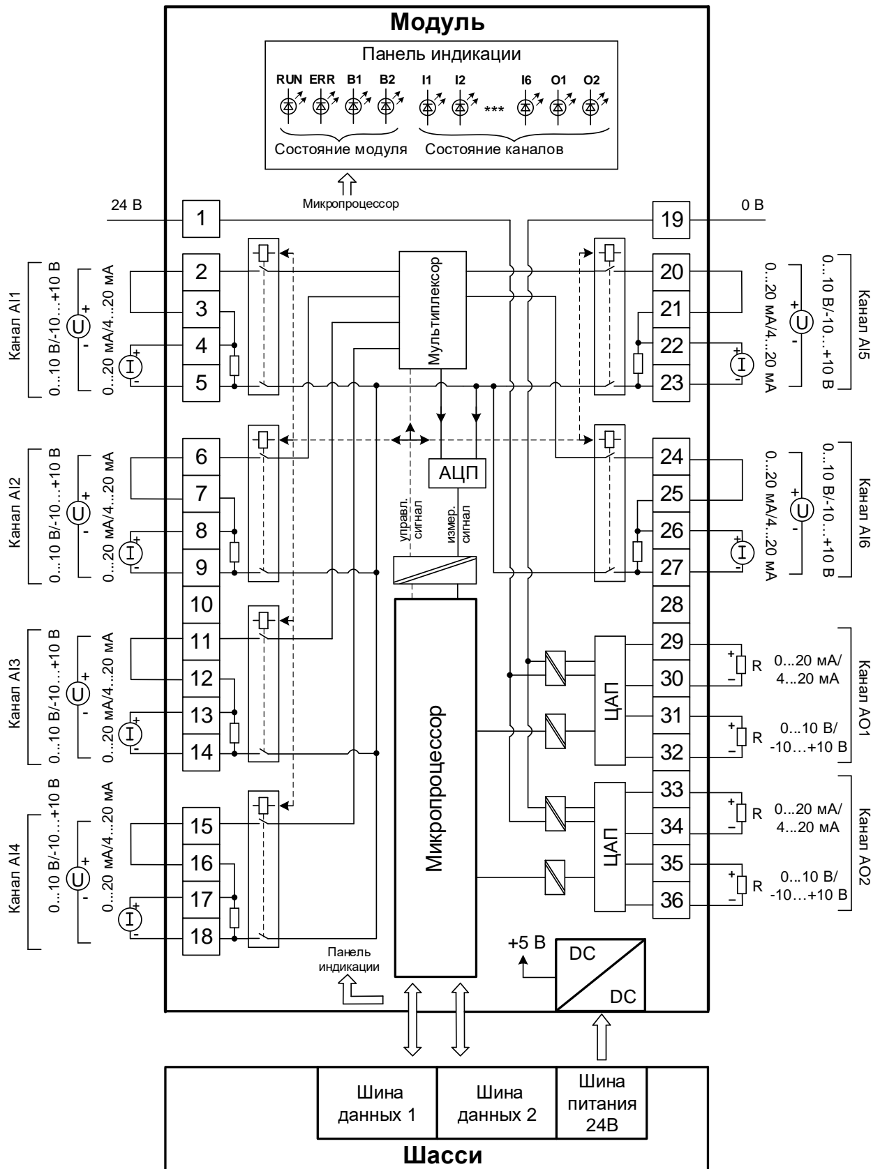
Рисунок 62 - Структурная схема модуля AS 08 011
