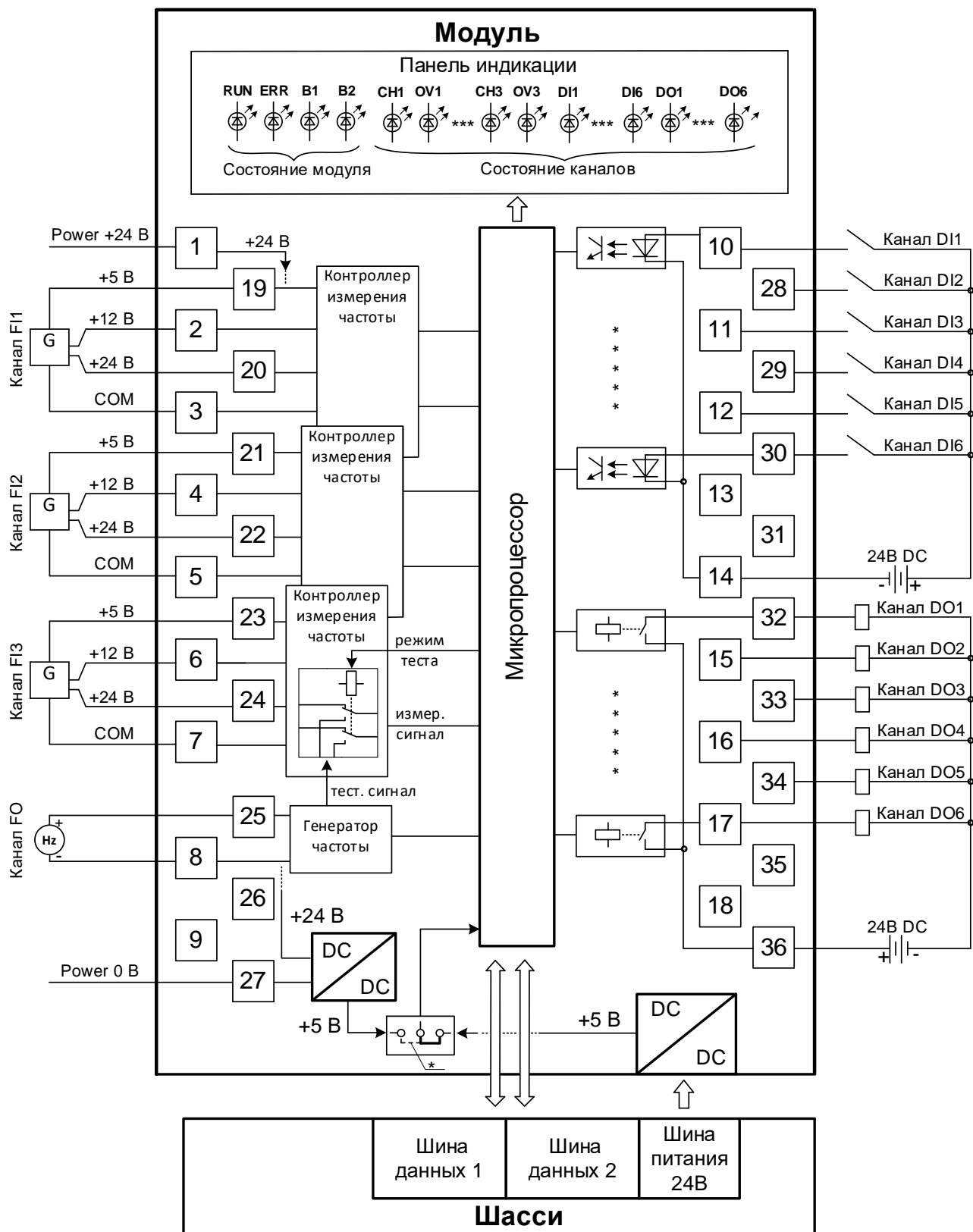
Рисунок 80 - Структурная схема модуля DA 03 021
