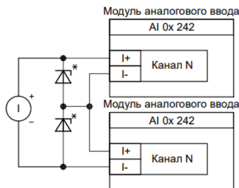
Рисунок В.8 - Подключение не резервированного датчика силы тока к резервированным каналам ввода аналоговых сигналов силы тока
