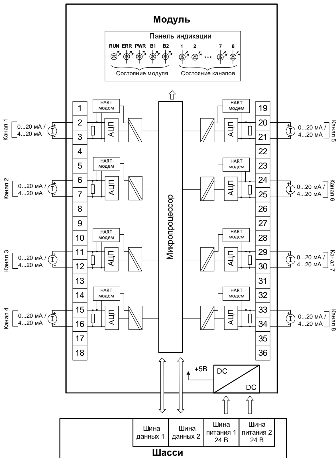
Рисунок 51 – Структурная схема модуля AI 08 022
