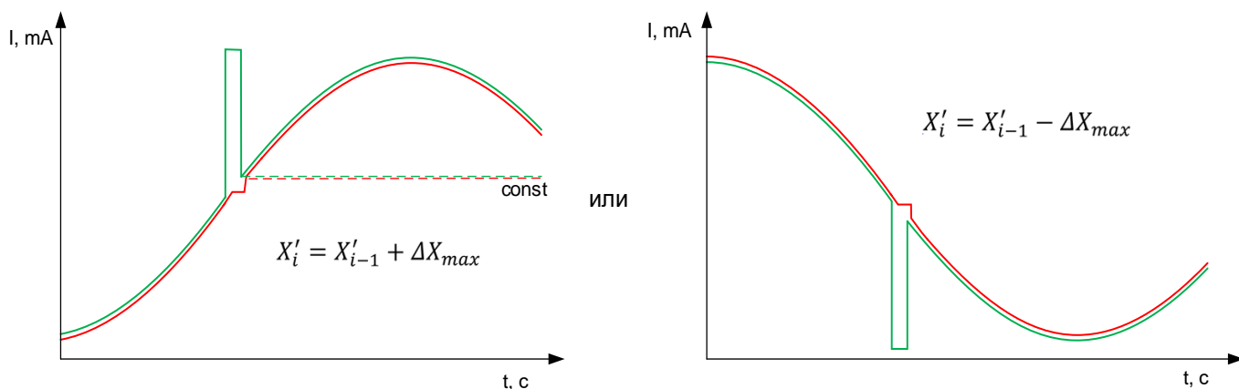
Рисунок 44 – Направление изменения величины X_i совпадает с направлением выброса
