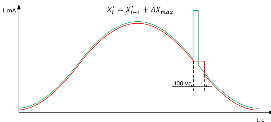
Рисунок 45 – Направление изменение величины X_i не совпадает с направлением выброса
