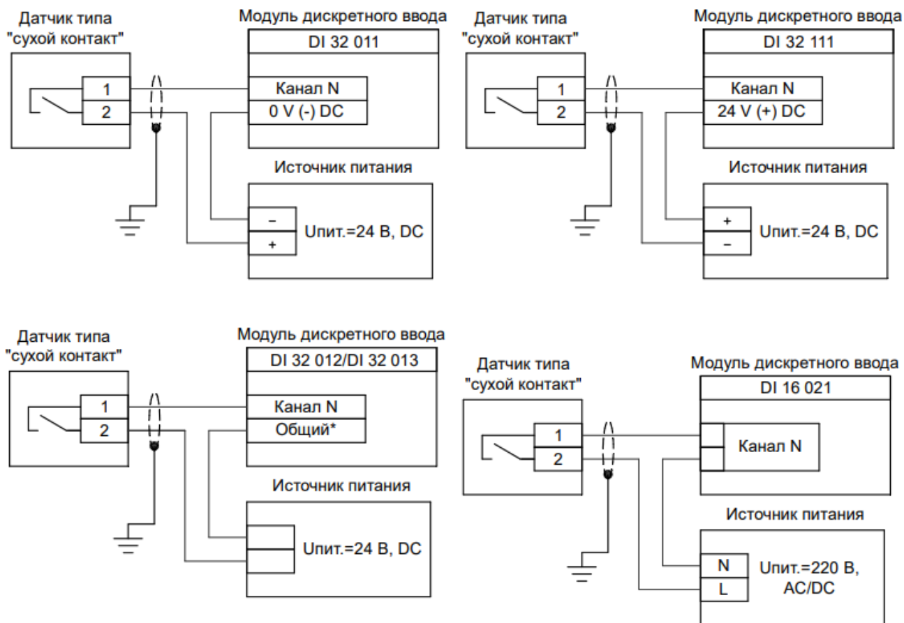
Рисунок Б.1.1 – Двухпроводные схемы подключения датчика типа «сухой контакт» к модулям дискретного ввода (*- не зависит от полярности приложенного напряжения)
