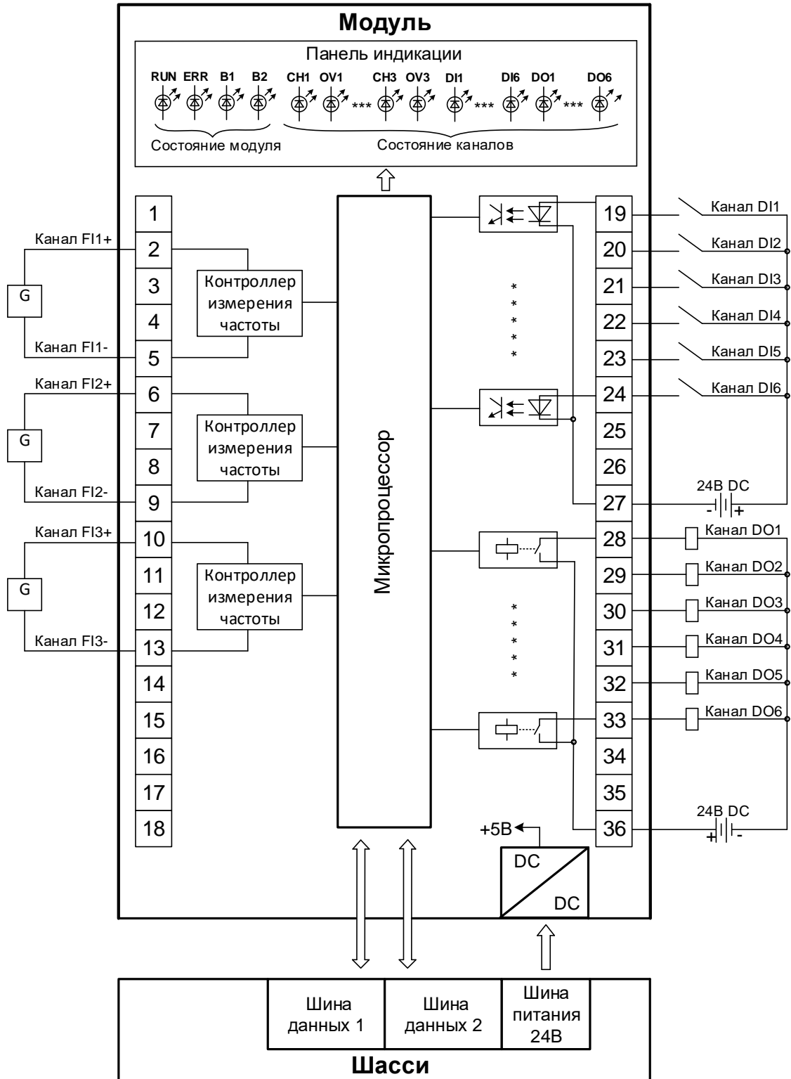
Рисунок 79 - Структурная схема модуля DA 03 011
