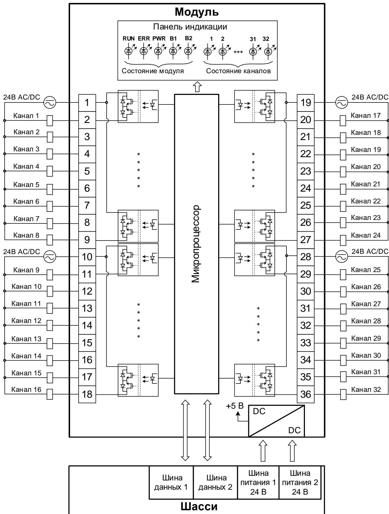
Рисунок 69 - Структурная схема модулей DO 32 012, DO 32 013
